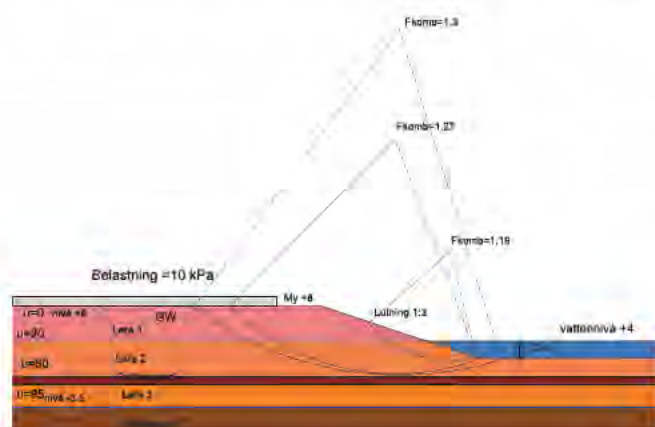
Figur 9-9. Exempel på en typslännt av lera med inlagrat skikt av friktionsjord som beräknats för nya klimatförutsättningar. (Hultén, 2005). I figuren visas stabilitetsförhållandena för dagens förhållanden.
