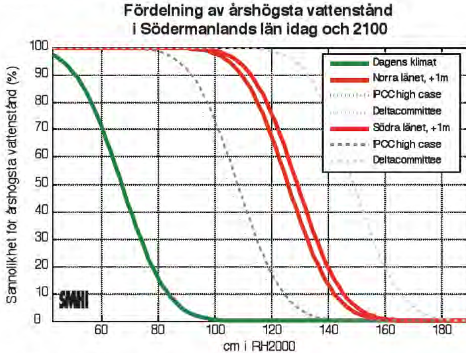
Figur 7-3. Sannolikhetsfördelning av årshögsta vattenstånd för Södermanlands län 2010, 2100 och 2200 i RH2000. Figuren visar hur extremerna förändras i ett klimat med stigande havsnivåer.
