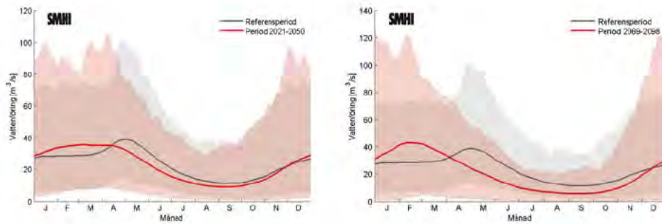
Figur 6-1. Säsongsdynamik för vattenföring i Eskilstunaån, baserat på klimatscenarier i Bilaga 1. Vänstra figuren är 2021-2050 jämfört med referensperioden 1963-1992. Högra figuren motsvarande för år 2069-2098. Heldragen svart linje visar medeltillrinning för referensperioden och heldragen röd linje visar medeltillrinning för den framtida tidsperioden. Det grå fältet visar variationen mellan 75:e percentilen av ensemblens maxvärde och 25:e percentilen av ensemblens minvärde under referensperioden. Det ljusröda fältet visar motsvarande för de framtida tidsperioderna.
