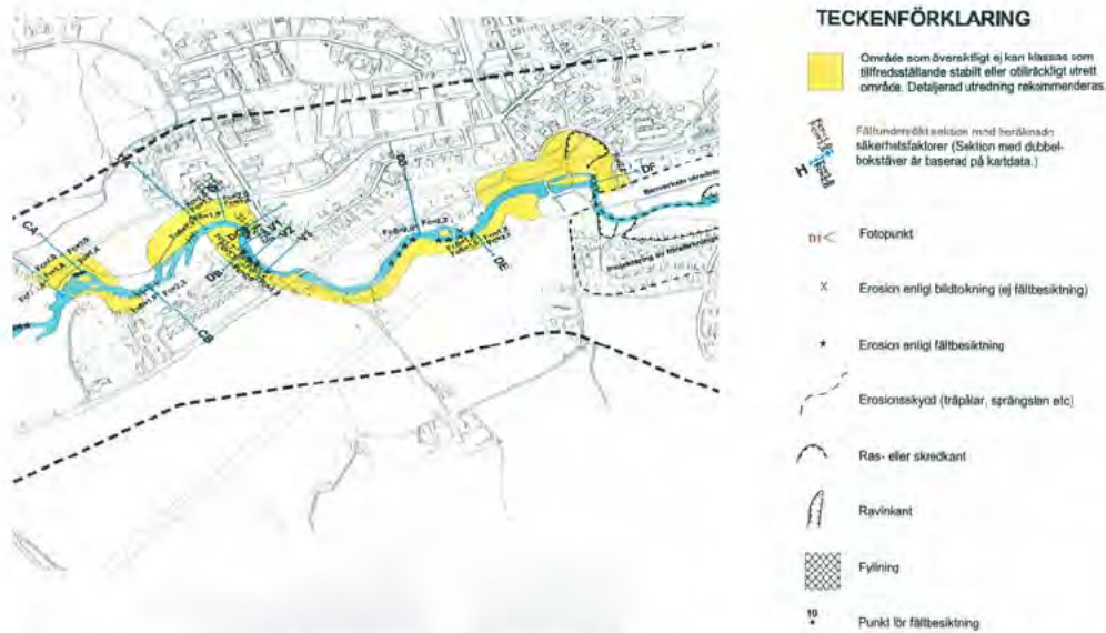
Figur 9-6. Exempel på redovisning av MSB:s översiktliga stabilitetskartering från Vagnhärad i Trosa kommun, Karta 1B (SGI,1997-11-24).
