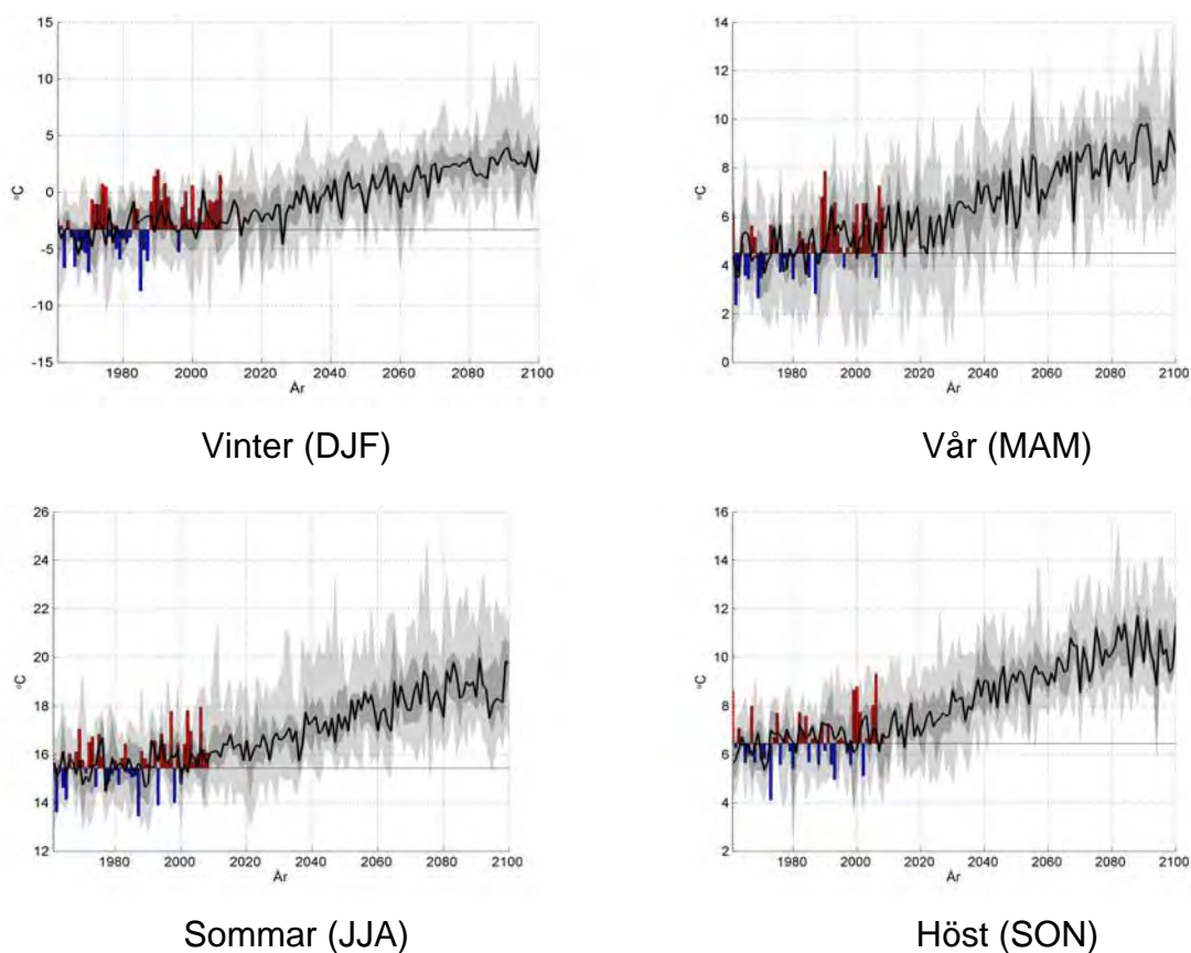
Figur 5-3. Beräknad temperaturutveckling i Södermanlands län för de olika årstiderna baserat på klimatscenarier i Bilaga 1. Historiska observationer visas som staplar. Observerade värden större än referensperiodens medelvärde visas som röda staplar och lägre värden visas som blå staplar. Skuggningarna avser uppifrån och nedåt, maximivärdet, 75:e percentilen, medianvärdet (svart linje), 25:e percentilen och minimivärdet av årsmedeltemperaturen från samtliga klimatberäkningar. Observera att skalan skiljer sig mellan figurerna.
