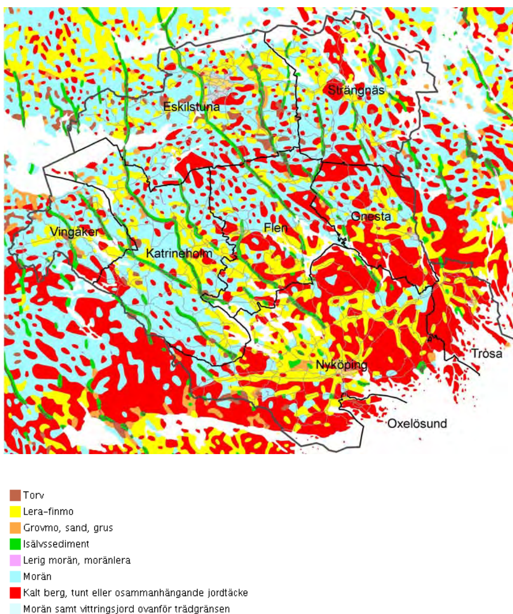
Figur 4-1. Översiktskarta över de geologiska förhållandena i Södermanlands län. Utdrag ur Sveriges jordarter – en översikt, WMS-tjänst från Sveriges Geologiska Undersökning, hämtad 2011-01-19.
