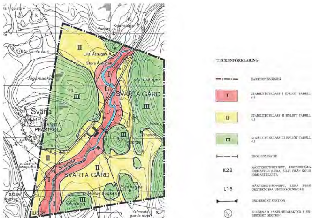
Figur 9-2. Exempel på redovisning av MSB:s översiktliga stabilitetskartering från Nyköpings kommun, Svärta, (VBB VIAC, 1993-04-30). Stabilitetszon I är markerad med röd färg.
