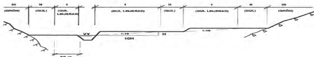
Figur 9-3 Kriterier för indelning och redovisning av stabilitetsförutsättningarna i lermark (MSB)
