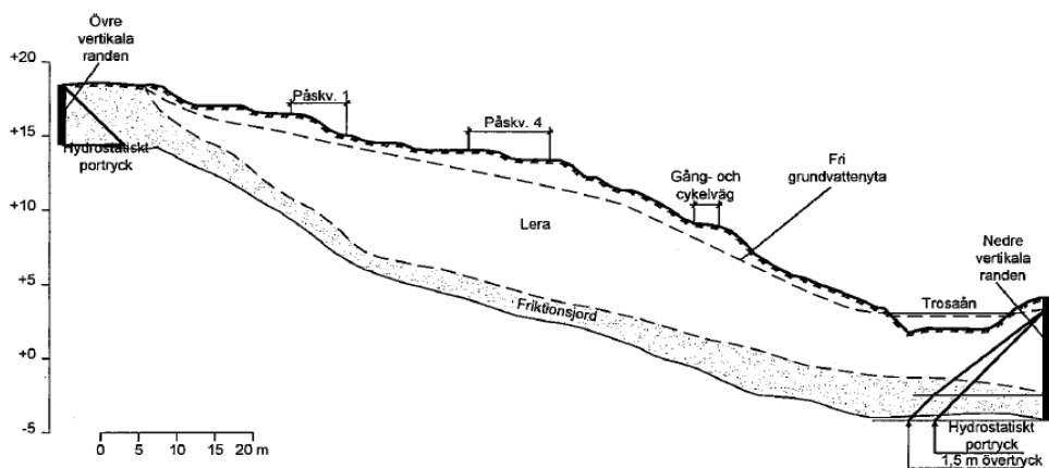
Figur 9-8 Geometri, jordarter och vattennivåer i sektionen genom initialscredet (Andersson et al, 1998)
