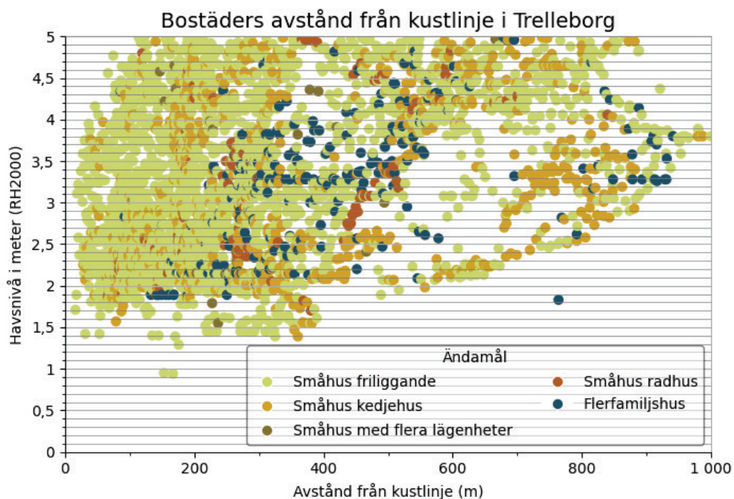
Figur 20 Samband mellan tröskelnivå för havsöversvämning, avstånd från kustlinjen upp till 1 km och ändamålet för bostadshus i Trelleborg kommun.
