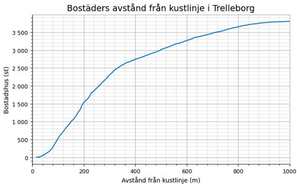
Figur 17 Antal bostadshus inom 1 km från kusten som översvämmas vid havsnivåer <5 m (RH2000) i Trelleborg kommun.
