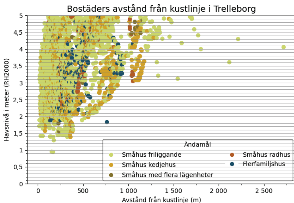
Figur 19 Samband mellan tröskelnivå för havsöversvämning, avstånd från kustlinjen och ändamålet för bostadshus i Trelleborg kommun. X-axelns utbredning bestäms av det maximala avståndet från kust till ett bostadshus som översvämmas vid <5 m (RH2000).
