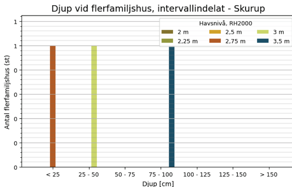
Figur 14 Samband i Skurup kommun mellan havsnivå och antalet flerfamiljshus som drabbas av översvämning, indelat i intervall för översvämningsdjup vid bostaden. Förutsätter att havsnivån varar tillräckligt länge för att maximalt potentiellt översvämningsdjup ska nås.
