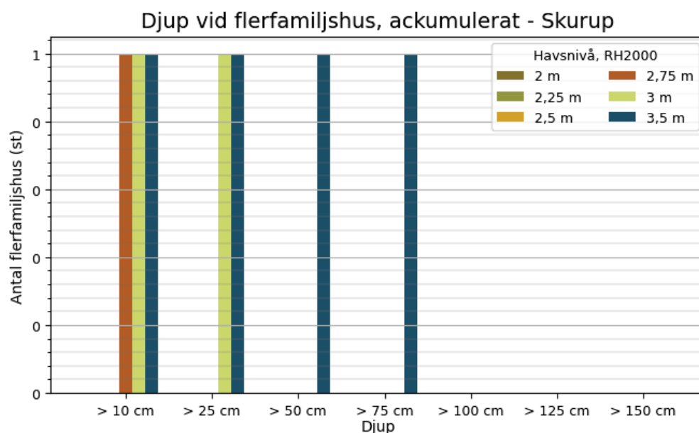
Figur 15 Samband i Skurup kommun mellan havsnivå och antalet flerfamiljshus som översvämmas med ett givet vattendjup eller mer. Förutsätter att havsnivån varar tillräckligt länge för att maximalt potentiellt översvämningsdjup ska hinna nås.
