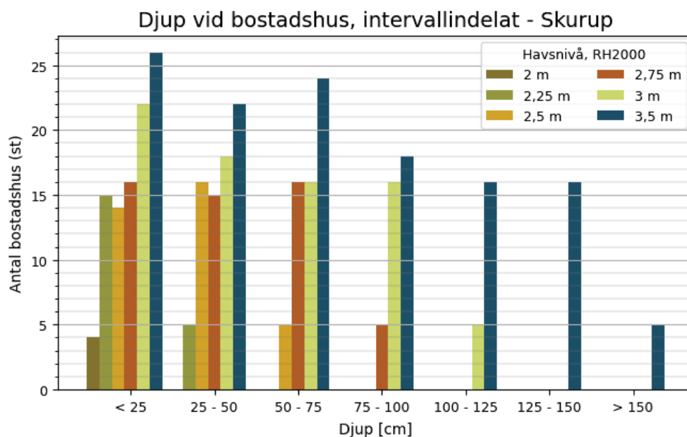
Figur 12 Samband i Skurup kommun mellan havsnivå och antalet bostadshus som drabbas av översvämning, indelat i intervall för översvämningsdjup vid bostad. Förutsätter att havsnivån varar tillräckligt länge för att maximalt potentiellt översvämningsdjup ska nås.
