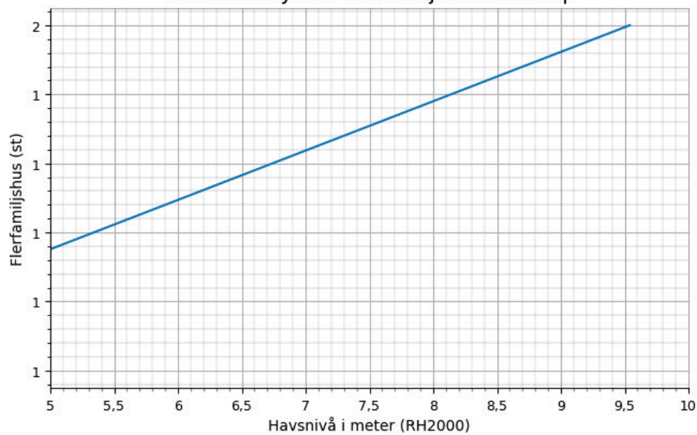
Figur 7 Antalet flerfamiljshus i Skurup kommun som riskerar att översvämmas vid havsnivåer mellan 5-10 m.
