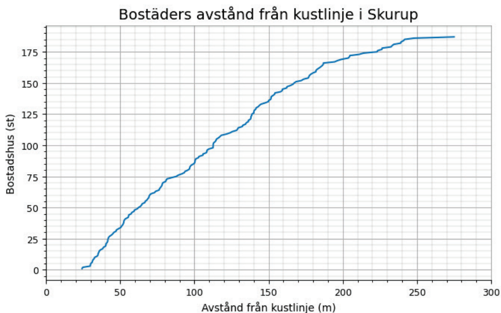
Figur 18 Antal bostadshus inom 300 m från kusten som översvämmas vid havsnivåer <5 m (RH2000) i Skurup kommun.
