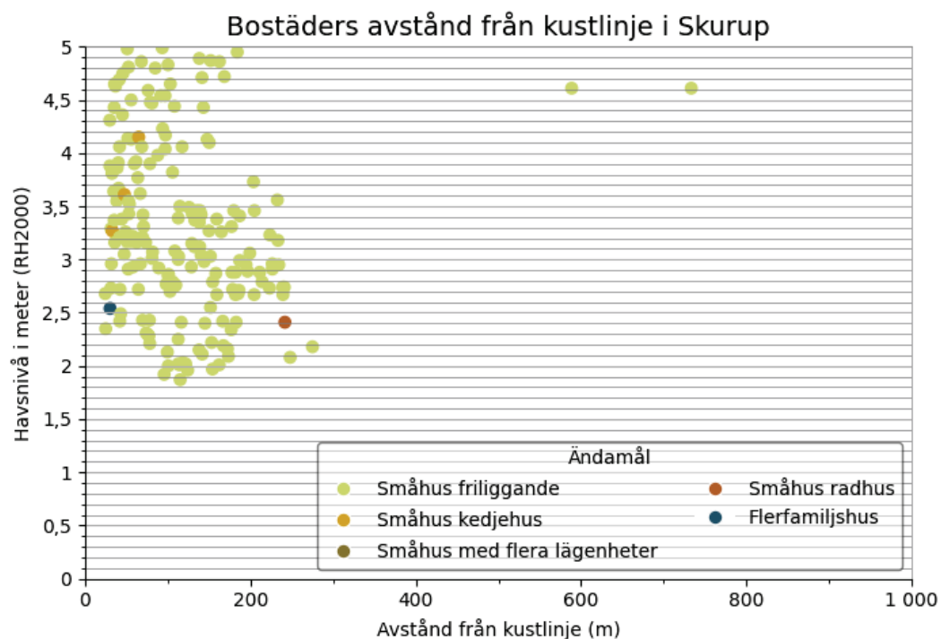
Figur 20 Samband mellan tröskelnivå för havsöversvämning, avstånd från kustlinjen upp till 1 km och ändamålet för bostadshus i Skurup kommun.
