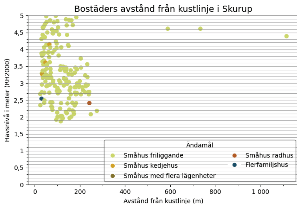
Figur 19 Samband mellan tröskelnivå för havsöversvämning, avstånd från kustlinjen och ändamålet för bostadshus i Skurup kommun. X-axelns utbredning bestäms av det maximala avståndet från kust till ett bostadshus som översvämmas vid <5 m (RH2000).
