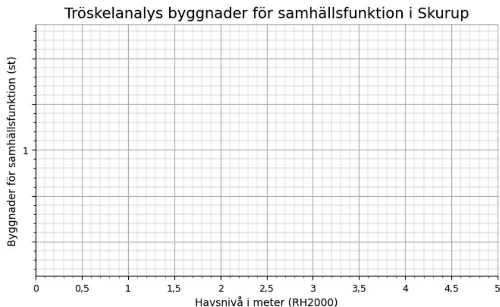
Figur 8 Antal byggnader för samhällsfunktion i Skurup kommun som riskerar att översvämmas vid havsnivåer mellan 0-5 m. De samhällsfunktioner som inkluderas i analysen är Sjukhus, Brandstation, Vårdcentral, Kommunhus och Polisstation.
