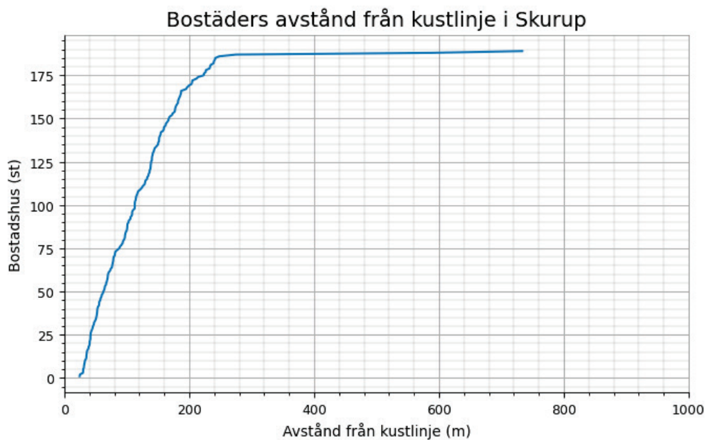
Figur 17 Antal bostadshus inom 1 km från kusten som översvämmas vid havsnivåer <5 m (RH2000) i Skurup kommun.
