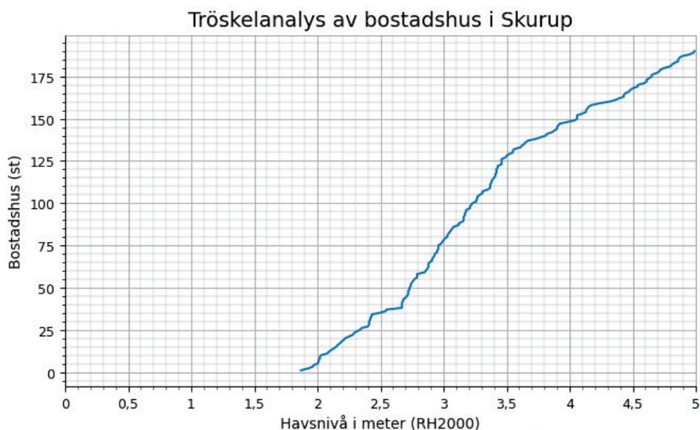
Figur 4 Antalet bostadshus i Skurup kommun som riskerar att översvämmas vid havsnivåer mellan 0-5 m. Bostadshus kan delas in i följande ändamål: Småhus friliggande, Småhus kedjehus, Småhus radhus, Småhus med flera lägenheter och Flerfamiljshus.
