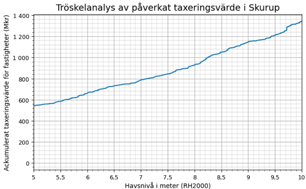
Figur 11 Det ackumulerade taxerade värdet (år 2023) för bostäder i Skurup kommun som riskerar att översvämmas vid havsnivåer mellan 5-10 m. Taxeringsvärdet inkluderar både tomtvärde och byggnadsvärde.
