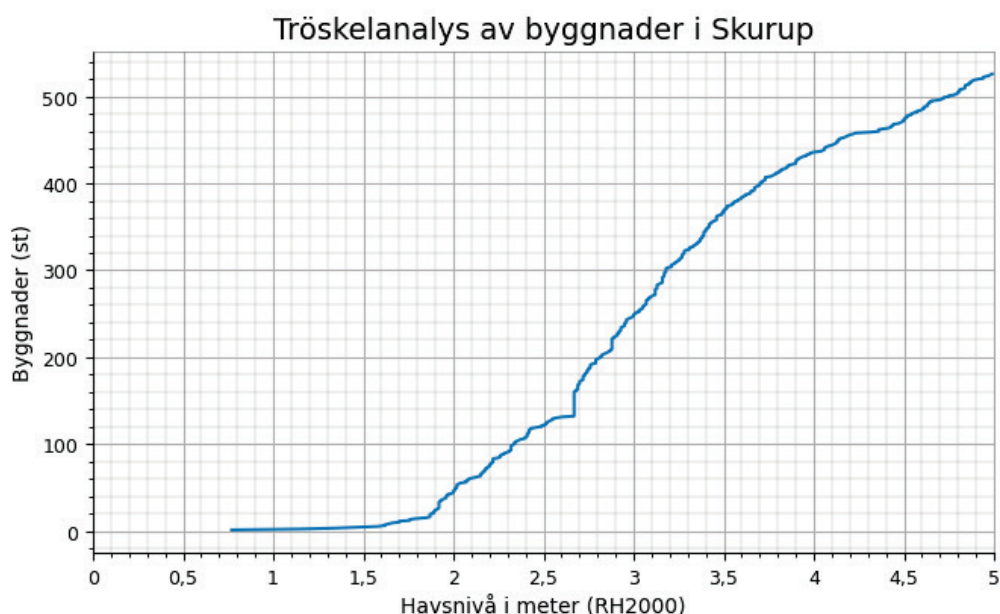
Figur 3 Antalet byggnader i Skurup kommun som riskerar att översvämmas vid havsnivåer mellan 0-5 m. Byggnader består av följande objektstyper: Bostad, Industri, Samhällsfunktion, Verksamhet, Ekonomibyggnad, Komplementbyggnad och Övrig byggnad.
