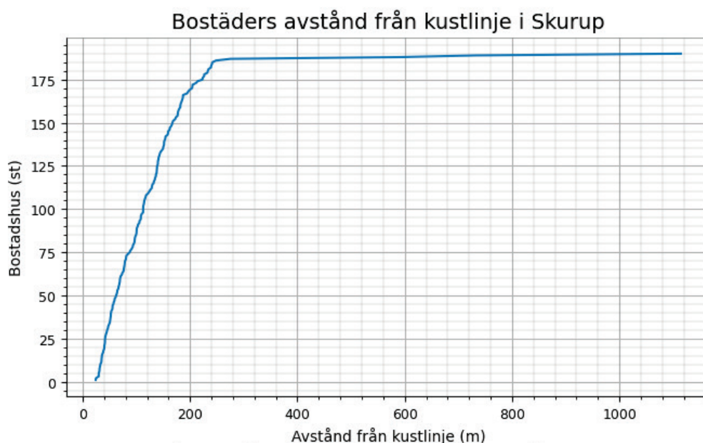
Figur 16 Antal bostadshus på givet avstånd från kusten som översvämmas vid havsnivåer <5 m (RH2000) i Skurup kommun. X-axelns utbredning bestäms av det maximala avståndet från kustlinjen till ett bostadshus som översvämmas vid <5 m (RH2000).
