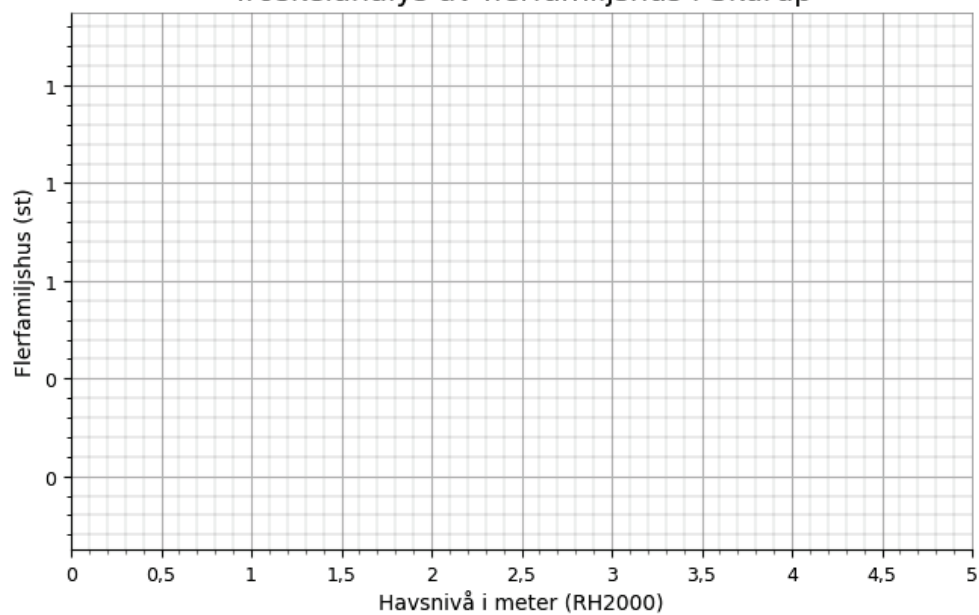
Figur 6 Antalet flerfamiljshus i Skurup kommun som riskerar att översvämmas vid havsnivåer mellan 0-5 m.
