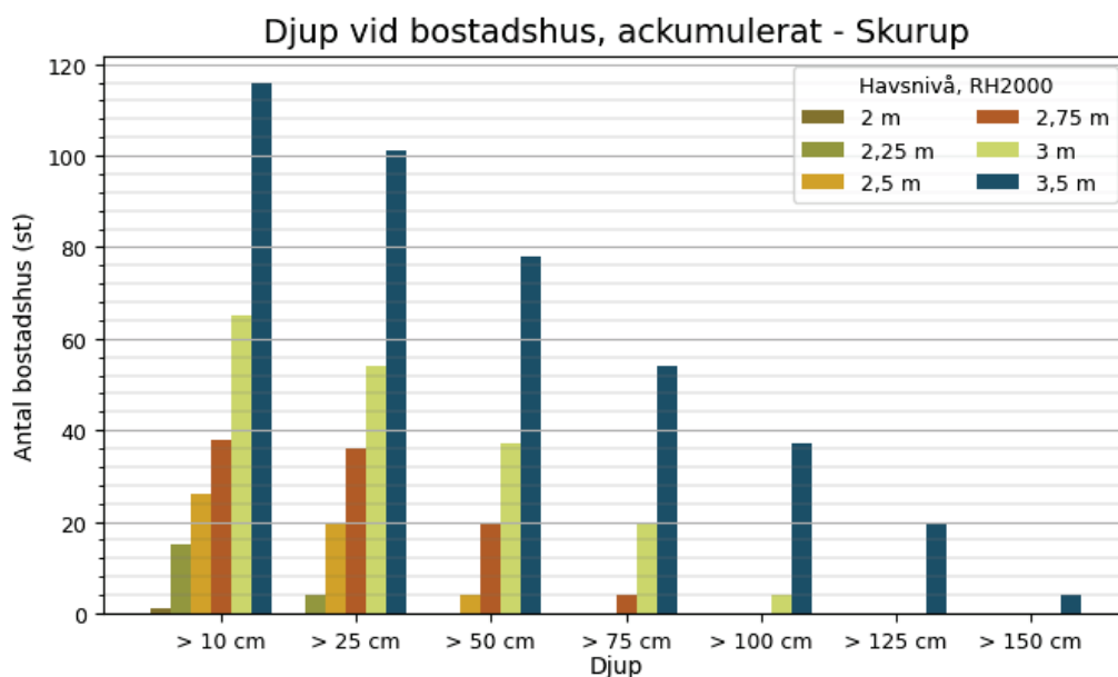
Figur 13 Samband i Skurup kommun mellan havsnivå och antalet bostadshus som översvämmas med ett givet vattendjup eller mer. Förutsätter att havsnivån varar tillräckligt länge för att maximalt potentiellt översvämningsdjup ska hinna nås.
