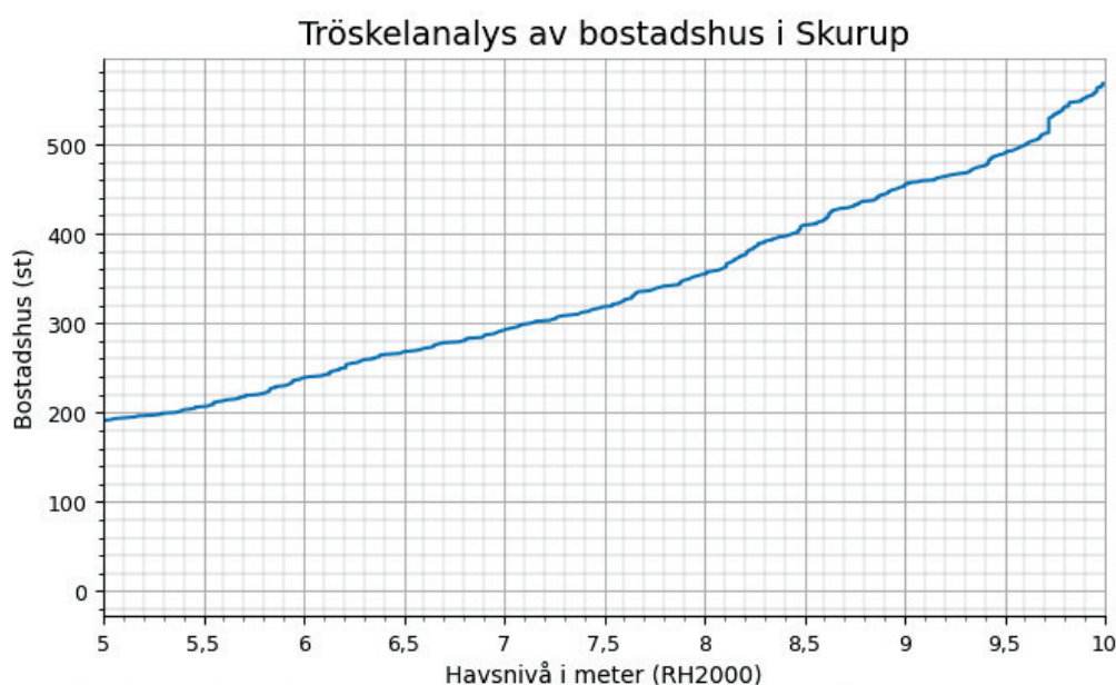
Figur 5 Antalet bostadshus i Skurup kommun som riskerar att översvämmas vid havsnivåer mellan 5-10 m. Bostadshus kan delas in i följande ändamål: Småhus friliggande, Småhus kedjehus, Småhus radhus, Småhus med flera lägenheter och Flerfamiljshus.
