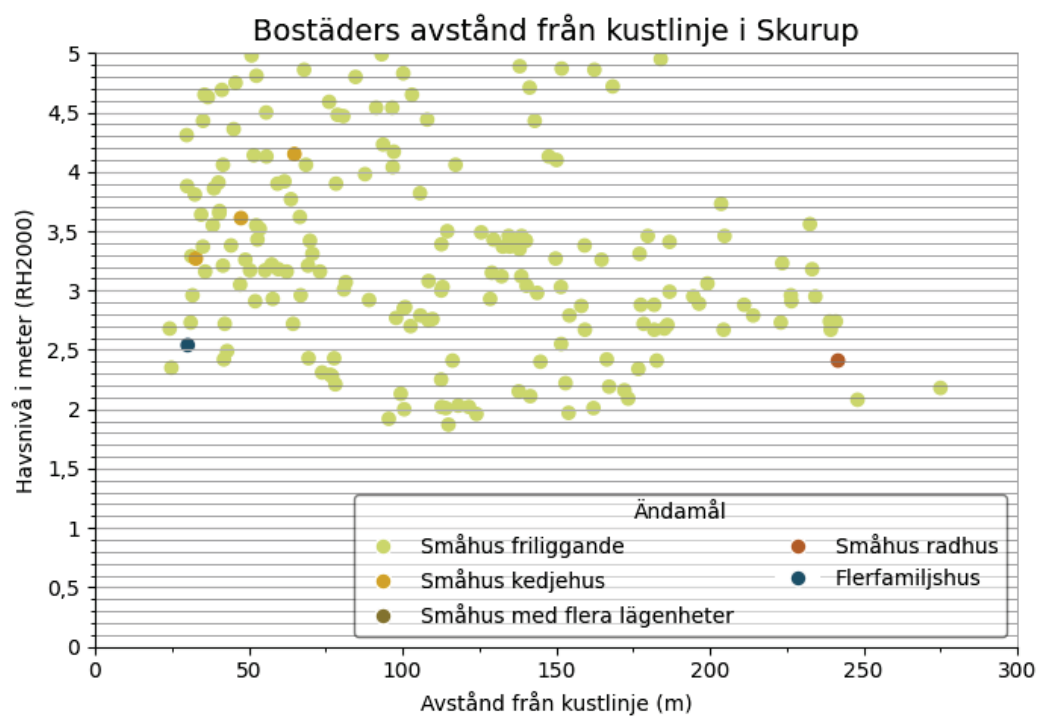
Figur 21 Samband mellan tröskelnivå för havsöversvämning, avstånd från kustlinjen upp till 300 m och ändamålet för bostadshus i Skurup kommun.
