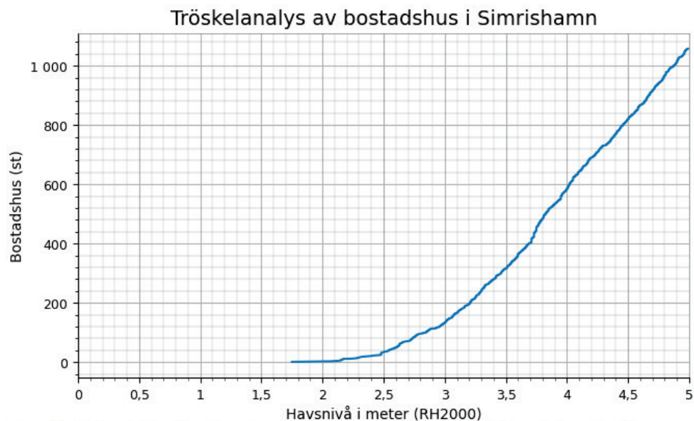
Figur 4 Antalet bostadshus i Simrishamn kommun som riskerar att översvämmas vid havsnivåer mellan 0-5 m. Bostadshus kan delas in i följande ändamål: Småhus friliggande, Småhus kedjehus, Småhus radhus, Småhus med flera lägenheter och Flerfamiljshus.
