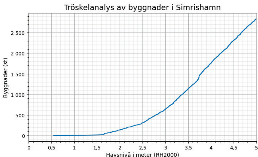
Figur 3 Antalet byggnader i Simrishamn kommun som riskerar att översvämmas vid havsnivåer mellan 0-5 m. Byggnader består av följande objektstyper: Bostad, Industri, Samhällsfunktion, Verksamhet, Ekonomibyggnad, Komplementbyggnad och Övrig byggnad.
