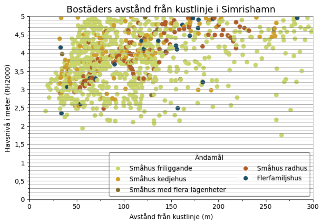
Figur 21 Samband mellan tröskelnivå för havsöversvämning, avstånd från kustlinjen upp till 300 m och ändamålet för bostadshus i Simrishamn kommun.
