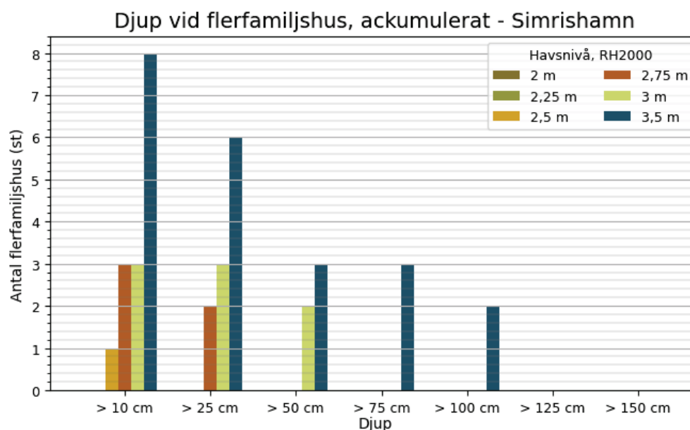
Figur 15 Samband i Simrishamn kommun mellan havsnivå och antalet flerfamiljshus som översvämmas med ett givet vattendjup eller mer. Förutsätter att havsnivån varar tillräckligt länge för att maximalt potentiellt översvämningsdjup ska hinna nås.
