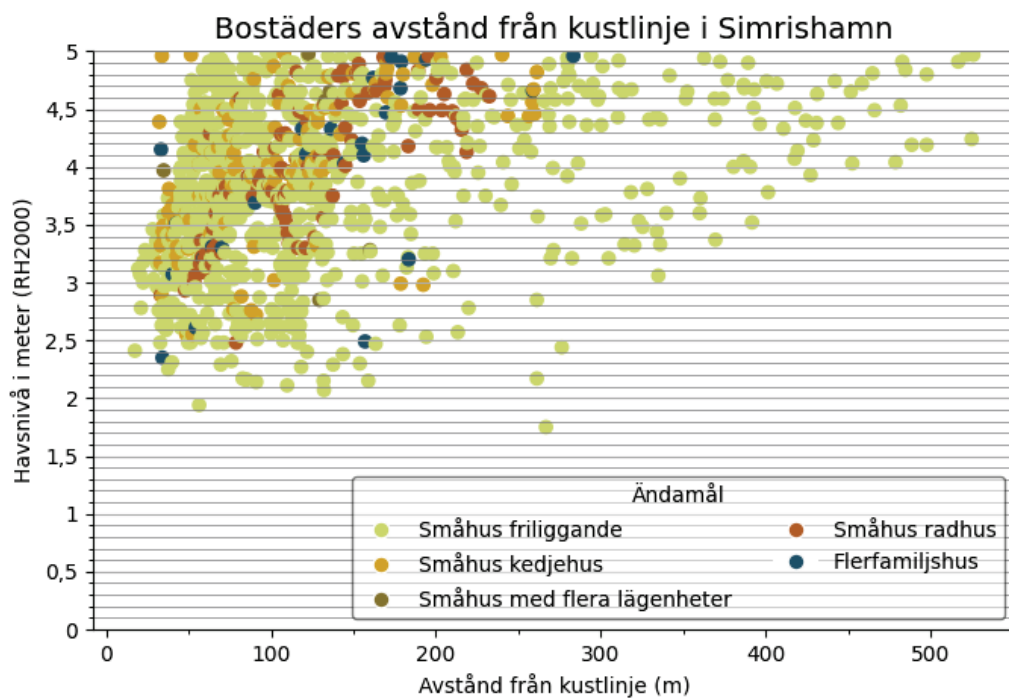
Figur 19 Samband mellan tröskelnivå för havsöversvämning, avstånd från kustlinjen och ändamålet för bostadshus i Simrishamn kommun. X-axelns utbredning bestäms av det maximala avståndet från kust till ett bostadshus som översvämmas vid <5 m (RH2000).
