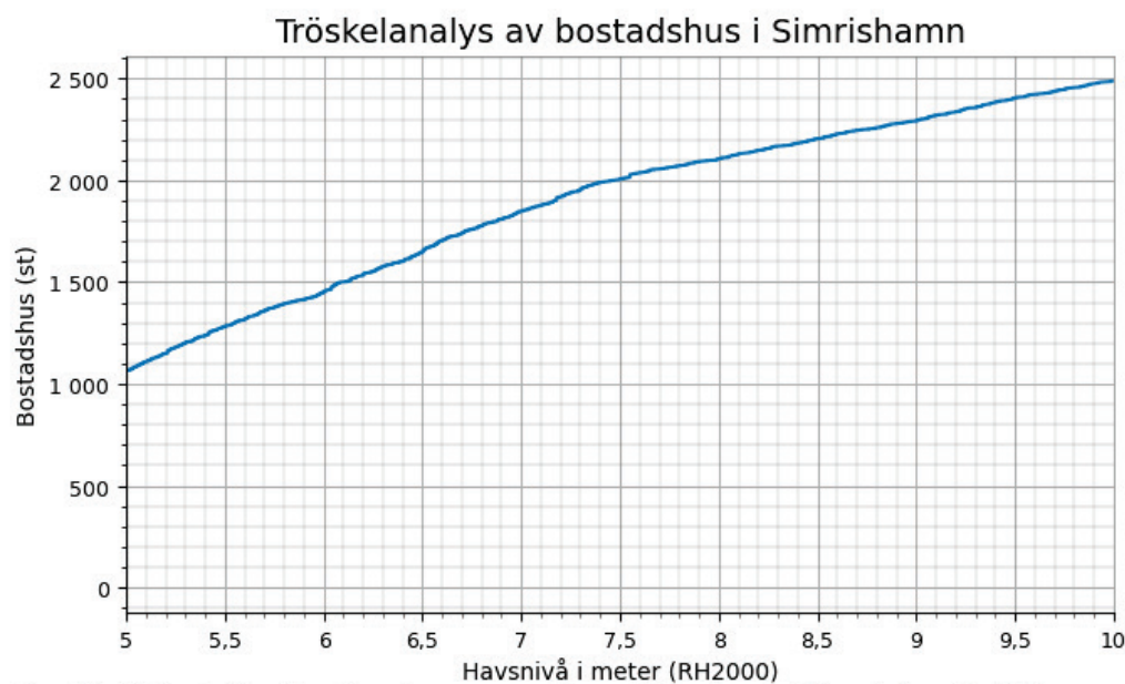
Figur 5 Antalet bostadshus i Simrishamn kommun som riskerar att översvämmas vid havsnivåer mellan 5-10 m. Bostadshus kan delas in i följande ändamål: Småhus friliggande, Småhus kedjehus, Småhus radhus, Småhus med flera lägenheter och Flerfamiljshus.
