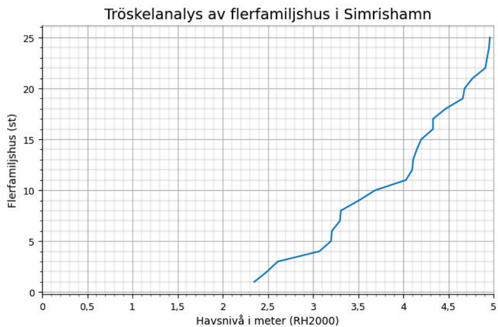
Figur 6 Antalet flerfamiljshus i Simrishamn kommun som riskerar att översvämmas vid havsnivåer mellan 0-5 m.
