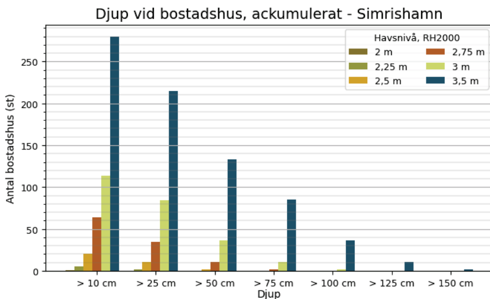
Figur 13 Samband i Simrishamn kommun mellan havsnivå och antalet bostadshus som översvämmas med ett givet vattendjup eller mer. Förutsätter att havsnivån varar tillräckligt länge för att maximalt potentiellt översvämningsdjup ska hinna nås.
