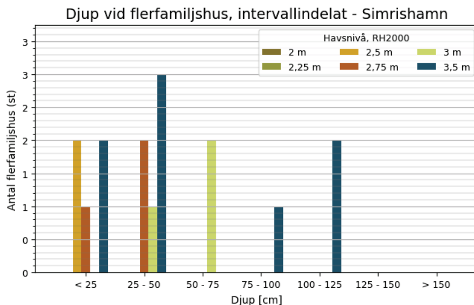
Figur 14 Samband i Simrishamn kommun mellan havsnivå och antalet flerfamiljshus som drabbas av översvämning, indelat i intervall för översvämningsdjup vid bostaden. Förutsätter att havsnivån varar tillräckligt länge för att maximalt potentiellt översvämningsdjup ska nås.
