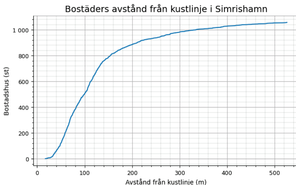
Figur 16 Antal bostadshus på givet avstånd från kusten som översvämmas vid havsnivåer <5 m (RH2000) i Simrishamn kommun. X-axelns utbredning bestäms av det maximala avståndet från kustlinjen till ett bostadshus som översvämmas vid <5 m (RH2000).
