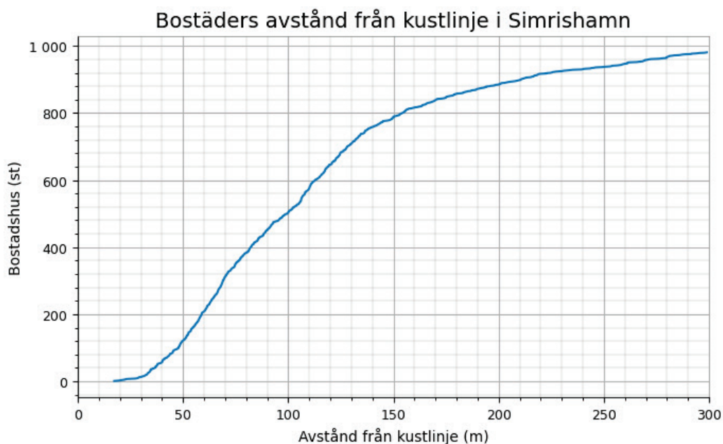
Figur 18 Antal bostadshus inom 300 m från kusten som översvämmas vid havsnivåer <5 m (RH2000) i Simrishamn kommun.
