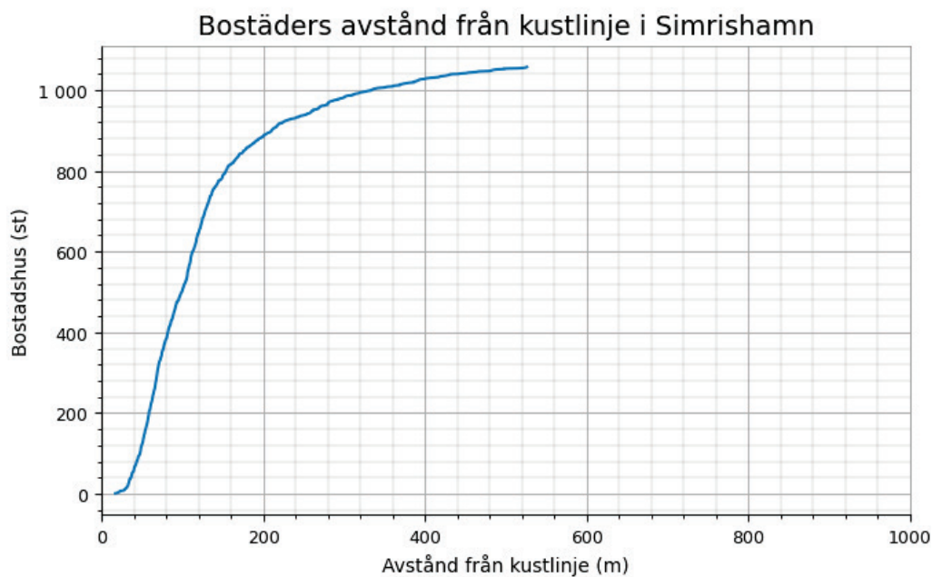
Figur 17 Antal bostadshus inom 1 km från kusten som översvämmas vid havsnivåer <5 m (RH2000) i Simrishamn kommun.
