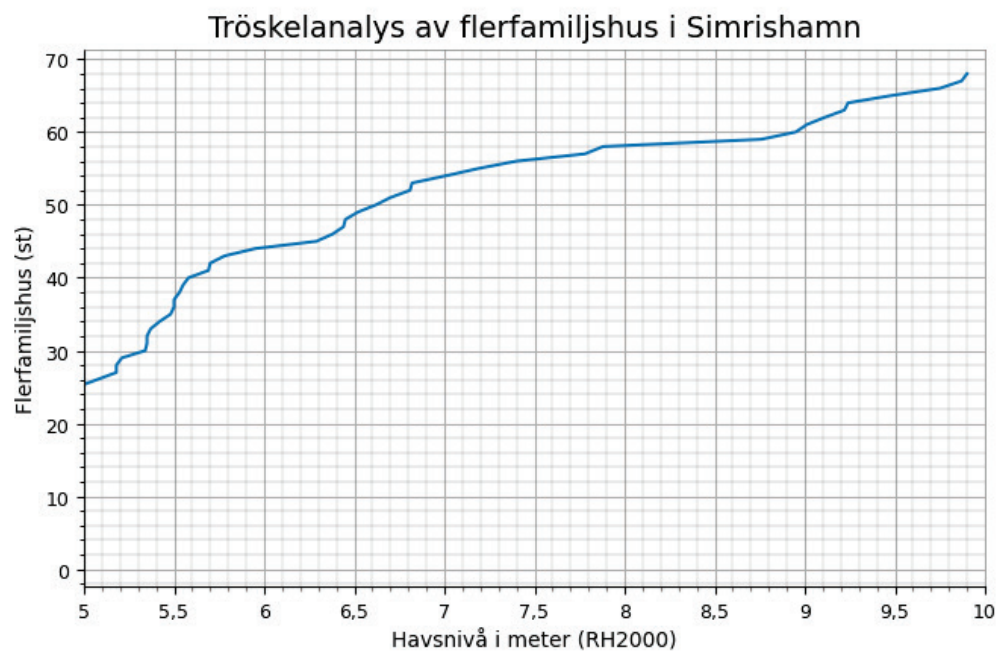
Figur 7 Antalet flerfamiljshus i Simrishamn kommun som riskerar att översvämmas vid havsnivåer mellan 5-10 m.
