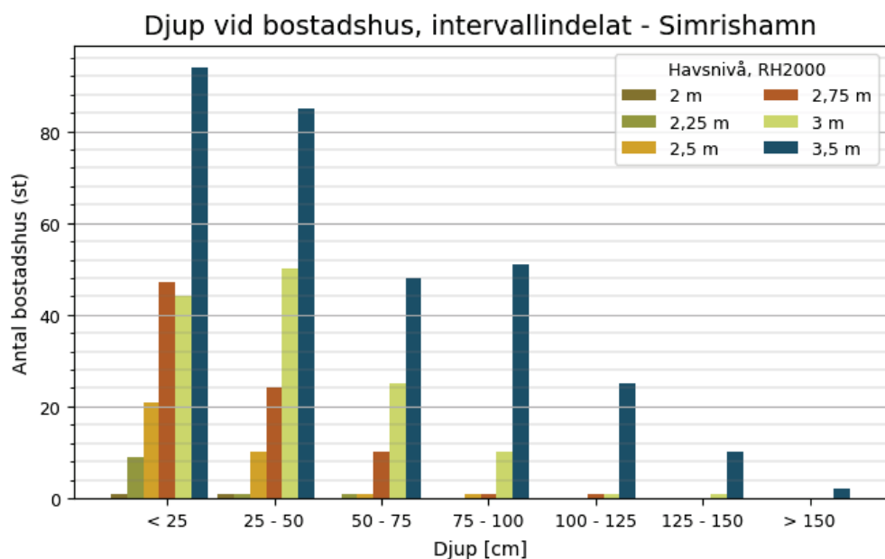
Figur 12 Samband i Simrishamn kommun mellan havsnivå och antalet bostadshus som drabbas av översvämning, indelat i intervall för översvämningsdjup vid bostad. Förutsätter att havsnivån varar tillräckligt länge för att maximalt potentiellt översvämningsdjup ska nås.
