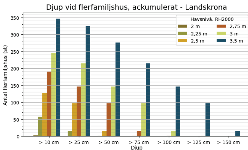
Figur 15 Samband i Landskrona kommun mellan havsnivå och antalet flerfamiljshus som översvämmas med ett givet vattendjup eller mer. Förutsätter att havsnivån varar tillräckligt länge för att maximalt potentiellt översvämningsdjup ska hinna nås.
