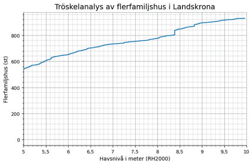
Figur 7 Antalet flerfamiljshus i Landskrona kommun som riskerar att översvämmas vid havsnivåer mellan 5-10 m.
