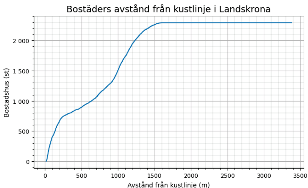
Figur 16 Antal bostadshus på givet avstånd från kusten som översvämmas vid havsnivåer <5 m (RH2000) i Landskrona kommun. X-axelns utbredning bestäms av det maximala avståndet från kustlinjen till ett bostadshus som översvämmas vid <5 m (RH2000).
