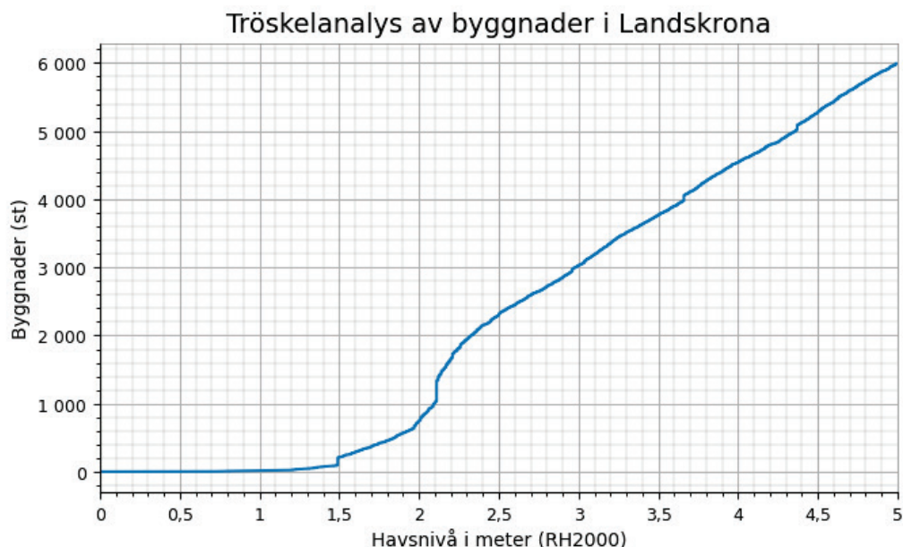
Figur 3 Antalet byggnader i Landskrona kommun som riskerar att översvämmas vid havsnivåer mellan 0-5 m. Byggnader består av följande objektstyper: Bostad, Industri, Samhällsfunktion, Verksamhet, Ekonomibyggnad, Komplementbyggnad och Övrig byggnad.
