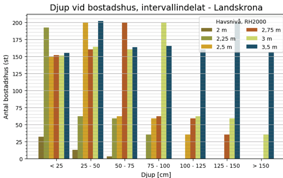
Figur 12 Samband i Landskrona kommun mellan havsnivå och antalet bostadshus som drabbas av översvämning, indelat i intervall för översvämningsdjup vid bostad. Förutsätter att havsnivån varar tillräckligt länge för att maximalt potentiellt översvämningsdjup ska nås.
