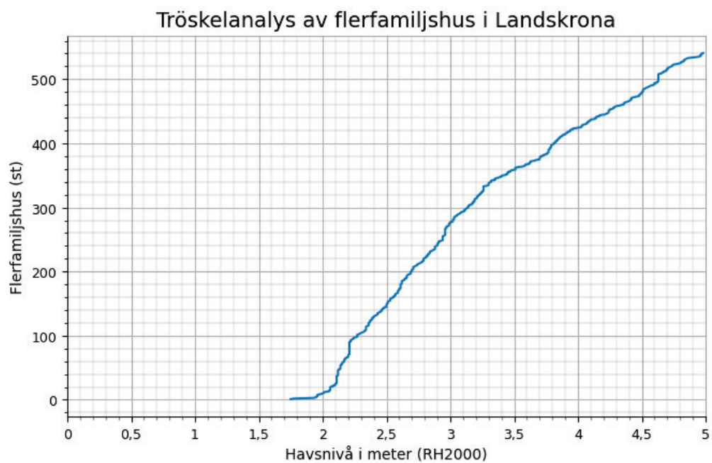
Figur 6 Antalet flerfamiljshus i Landskrona kommun som riskerar att översvämmas vid havsnivåer mellan 0-5 m.
