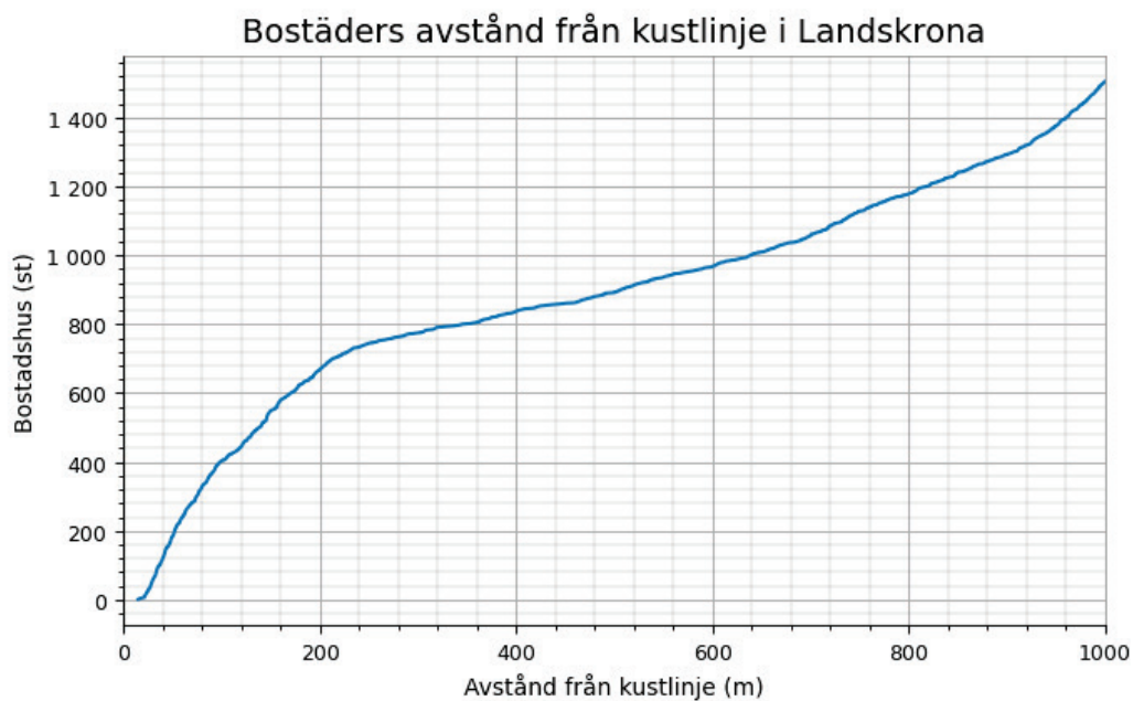
Figur 17 Antal bostadshus inom 1 km från kusten som översvämmas vid havsnivåer <5 m (RH2000) i Landskrona kommun.
