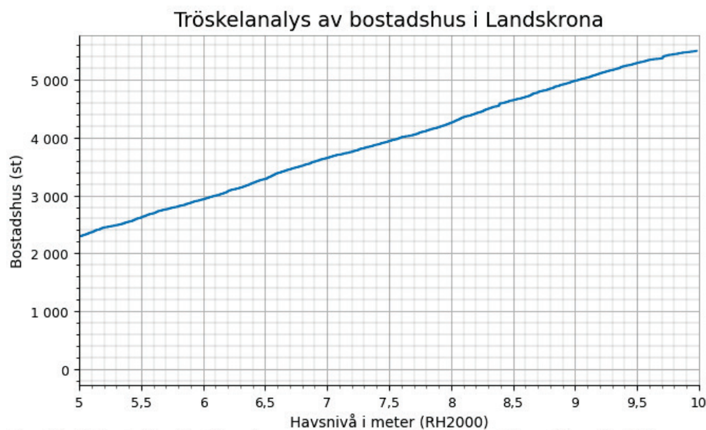
Figur 5 Antalet bostadshus i Landskrona kommun som riskerar att översvämmas vid havsnivåer mellan 5-10 m. Bostadshus kan delas in i följande ändamål: Småhus friliggande, Småhus kedjehus, Småhus radhus, Småhus med flera lägenheter och Flerfamiljshus.
