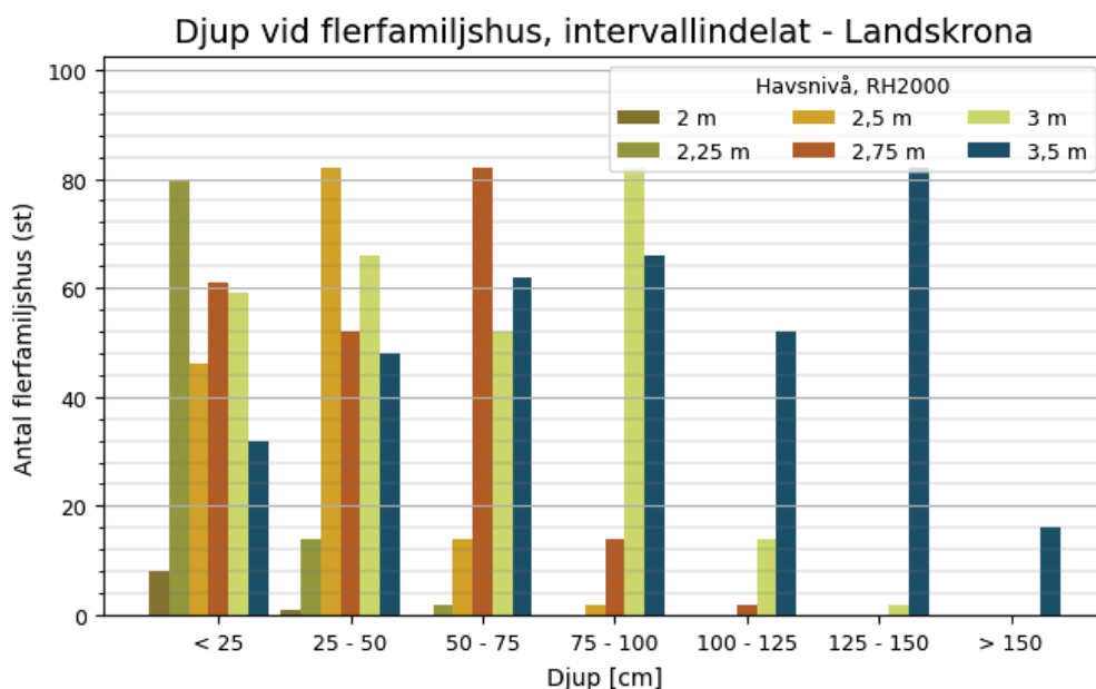
Figur 14 Samband i Landskrona kommun mellan havsnivå och antalet flerfamiljshus som drabbas av översvämning, indelat i intervall för översvämningsdjup vid bostaden. Förutsätter att havsnivån varar tillräckligt länge för att maximalt potentiellt översvämningsdjup ska nås.
