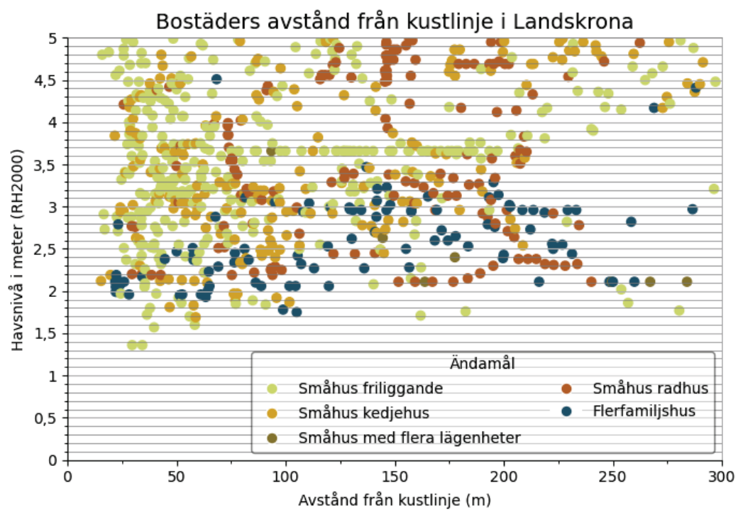
Figur 21 Samband mellan tröskelnivå för havsöversvämning, avstånd från kustlinjen upp till 300 m och ändamålet för bostadshus i Landskrona kommun.
