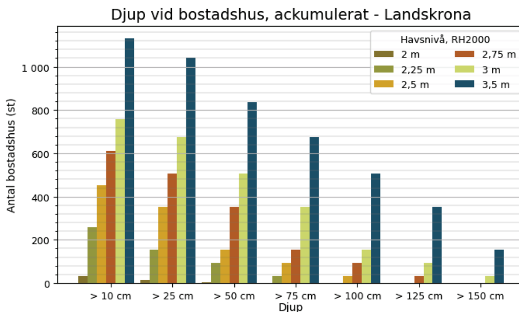
Figur 13 Samband i Landskrona kommun mellan havsnivå och antalet bostadshus som översvämmas med ett givet vattendjup eller mer. Förutsätter att havsnivån varar tillräckligt länge för att maximalt potentiellt översvämningsdjup ska hinna nås.
