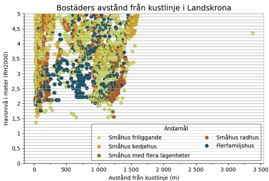
Figur 19 Samband mellan tröskelnivå för havsöversvämning, avstånd från kustlinjen och ändamålet för bostadshus i Landskrona kommun. X-axelns utbredning bestäms av det maximala avståndet från kust till ett bostadshus som översvämmas vid <5 m (RH2000).
