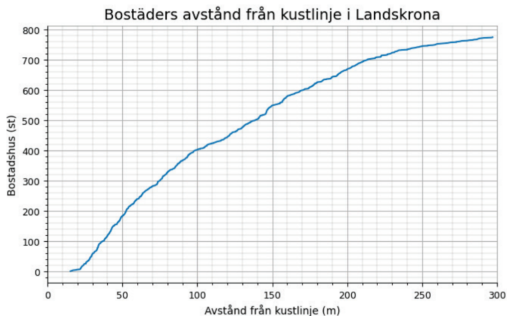
Figur 18 Antal bostadshus inom 300 m från kusten som översvämmas vid havsnivåer <5 m (RH2000) i Landskrona kommun.
