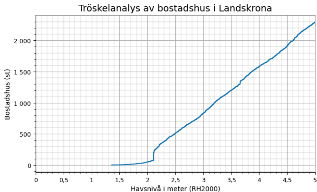
Figur 4 Antalet bostadshus i Landskrona kommun som riskerar att översvämmas vid havsnivåer mellan 0-5 m. Bostadshus kan delas in i följande ändamål: Småhus friliggande, Småhus kedjehus, Småhus radhus, Småhus med flera lägenheter och Flerfamiljshus.
