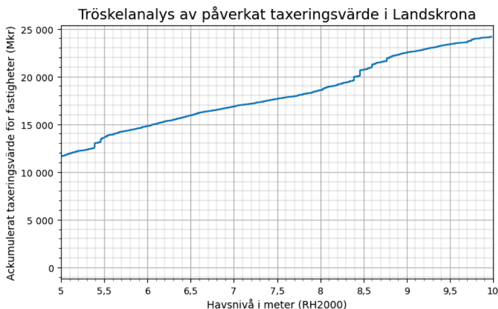
Figur 11 Det ackumulerade taxerade värdet (år 2023) för bostäder i Landskrona kommun som riskerar att översvämmas vid havsnivåer mellan 5-10 m. Taxeringsvärdet inkluderar både tomtvärde och byggnadsvärde.
