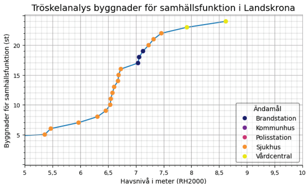
Figur 9 Antal byggnader för samhällsfunktion i Landskrona kommun som riskerar att översvämmas vid havsnivåer mellan 5-10 m. De samhällsfunktioner som inkluderas i analysen är Sjukhus, Brandstation, Vårdcentral, Kommunhus och Polisstation.
