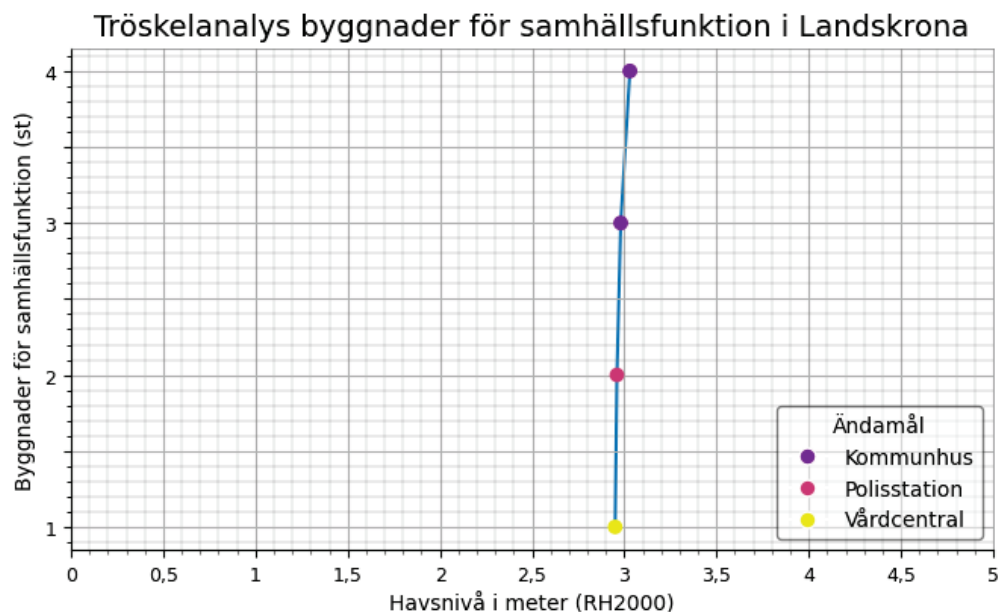
Figur 8 Antal byggnader för samhällsfunktion i Landskrona kommun som riskerar att översvämmas vid havsnivåer mellan 0-5 m. De samhällsfunktioner som inkluderas i analysen är Sjukhus, Brandstation, Vårdcentral, Kommunhus och Polisstation.
