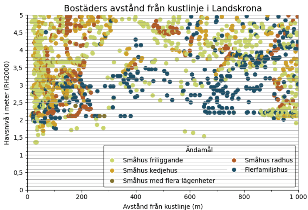
Figur 20 Samband mellan tröskelnivå för havsöversvämning, avstånd från kustlinjen upp till 1 km och ändamålet för bostadshus i Landskrona kommun.
