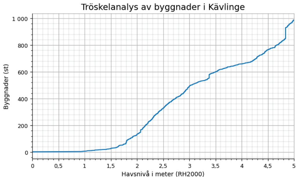
Figur 3 Antalet byggnader i Kävlinge kommun som riskerar att översvämmas vid havsnivåer mellan 0-5 m. Byggnader består av följande objektstyper: Bostad, Industri, Samhällsfunktion, Verksamhet, Ekonomibyggnad, Komplementbyggnad och Övrig byggnad.
