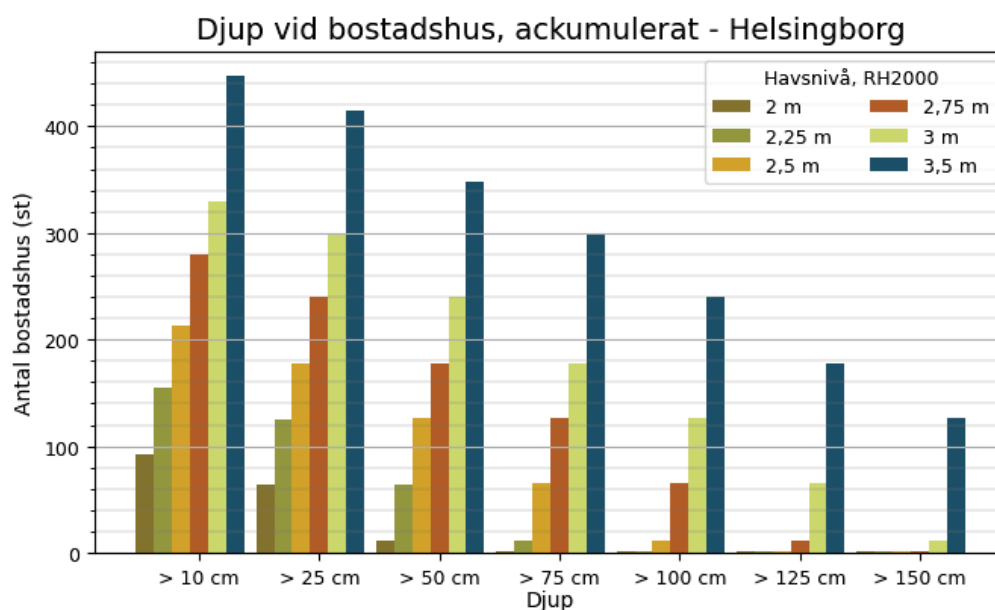
Figur 13 Samband i Helsingborg kommun mellan havsnivå och antalet bostadshus som översvämmas med ett givet vattendjup eller mer. Förutsätter att havsnivån varar tillräckligt länge för att maximalt potentiellt översvämningsdjup ska hinna nås.
