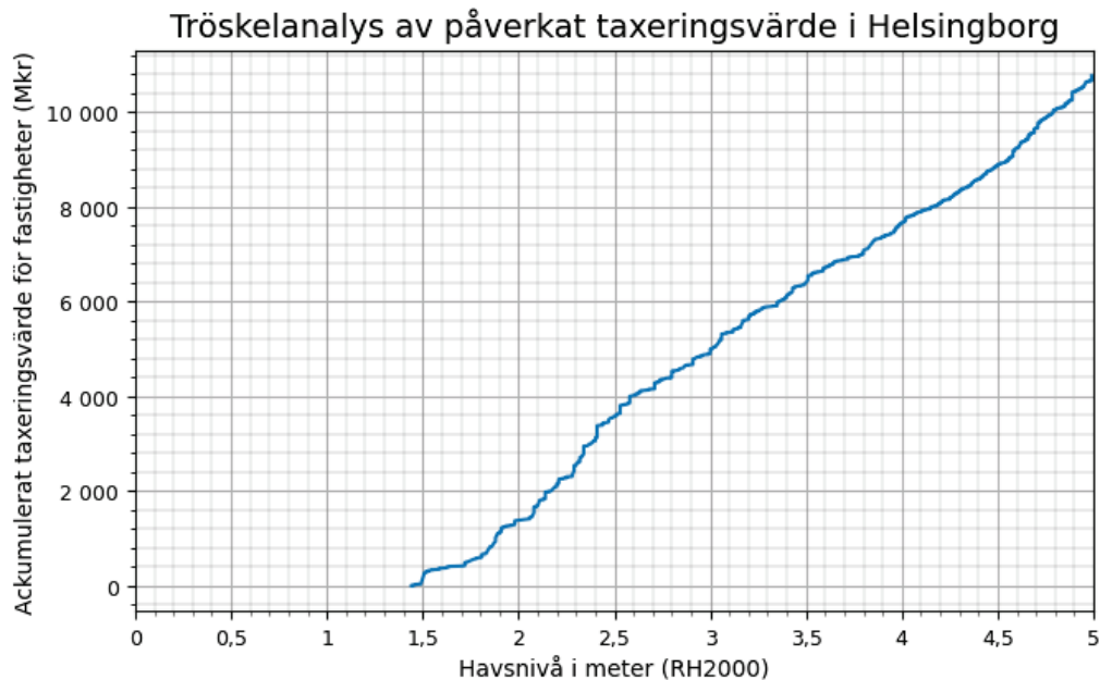
Figur 10 Det ackumulerade taxerade värdet (år 2023) för bostäder i Helsingborg kommun som riskerar att översvämmas vid havsnivåer mellan 0-5 m. Taxeringsvärdet inkluderar både tomtvärde och byggnadsvärde.
