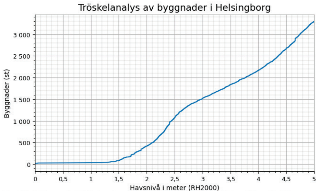
Figur 3 Antalet byggnader i Helsingborg kommun som riskerar att översvämmas vid havsnivåer mellan 0-5 m. Byggnader består av följande objektstyper: Bostad, Industri, Samhällsfunktion, Verksamhet, Ekonomibyggnad, Komplementbyggnad och Övrig byggnad.
