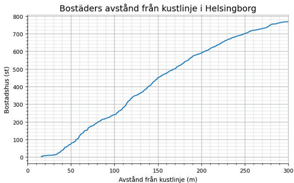
Figur 18 Antal bostadshus inom 300 m från kusten som översvämmas vid havsnivåer <5 m (RH2000) i Helsingborg kommun.
