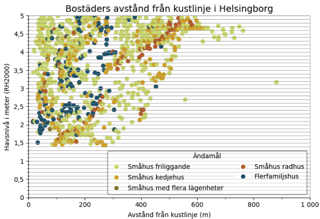
Figur 20 Samband mellan tröskelnivå för havsöversvämning, avstånd från kustlinjen upp till 1 km och ändamålet för bostadshus i Helsingborg kommun.
