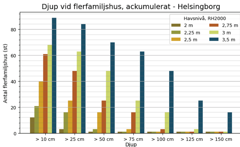
Figur 15 Samband i Helsingborg kommun mellan havsnivå och antalet flerfamiljshus som översvämmas med ett givet vattendjup eller mer. Förutsätter att havsnivån varar tillräckligt länge för att maximalt potentiellt översvämningsdjup ska hinna nås.
