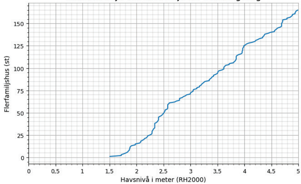
Figur 6 Antalet flerfamiljshus i Helsingborg kommun som riskerar att översvämmas vid havsnivåer mellan 0-5 m.
