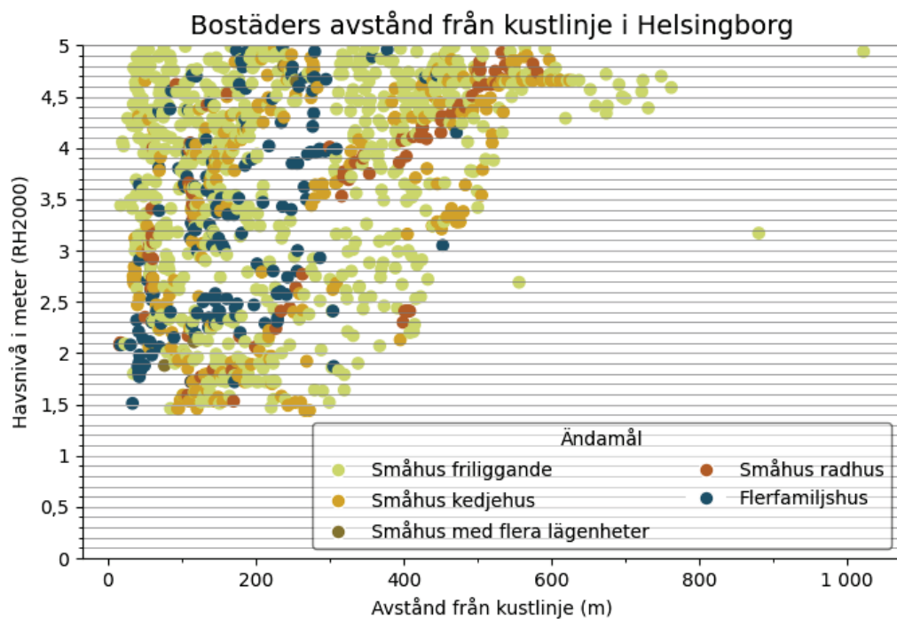
Figur 19 Samband mellan tröskelnivå för havsöversvämning, avstånd från kustlinjen och ändamålet för bostadshus i Helsingborg kommun. X-axelns utbredning bestäms av det maximala avståndet från kust till ett bostadshus som översvämmas vid <5 m (RH2000).
