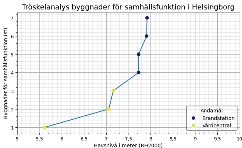
Figur 9 Antal byggnader för samhällsfunktion i Helsingborg kommun som riskerar att översvämmas vid havsnivåer mellan 5-10 m. De samhällsfunktioner som inkluderas i analysen är Sjukhus, Brandstation, Vårdcentral, Kommunhus och Polisstation.
