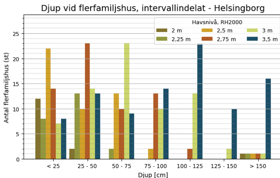
Figur 14 Samband i Helsingborg kommun mellan havsnivå och antalet flerfamiljshus som drabbas av översvämning, indelat i intervall för översvämningsdjup vid bostaden. Förutsätter att havsnivån varar tillräckligt länge för att maximalt potentiellt översvämningsdjup ska nås.
