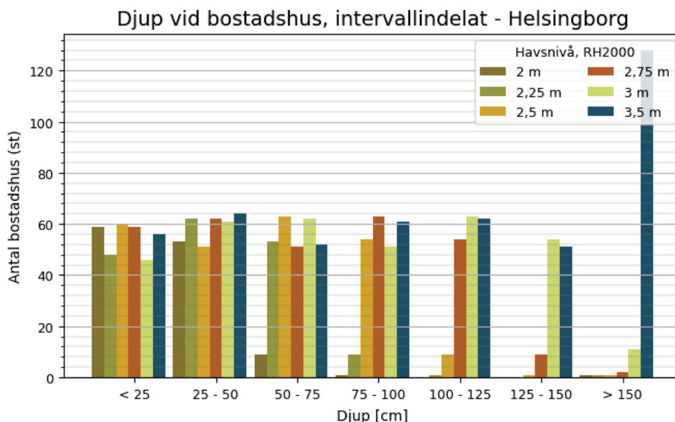
Figur 12 Samband i Helsingborg kommun mellan havsnivå och antalet bostadshus som drabbas av översvämnning, indelat i intervall för översvämningsdjup vid bostad. Förutsätter att havsnivån varar tillräckligt länge för att maximalt potentiellt översvämningsdjup ska nås.
