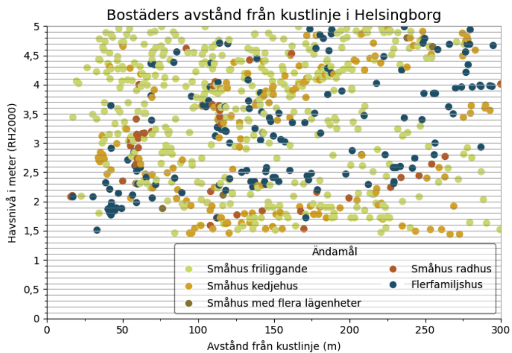
Figur 21 Samband mellan tröskelnivå för havsöversvämning, avstånd från kustlinjen upp till 300 m och ändamålet för bostadshus i Helsingborg kommun.
