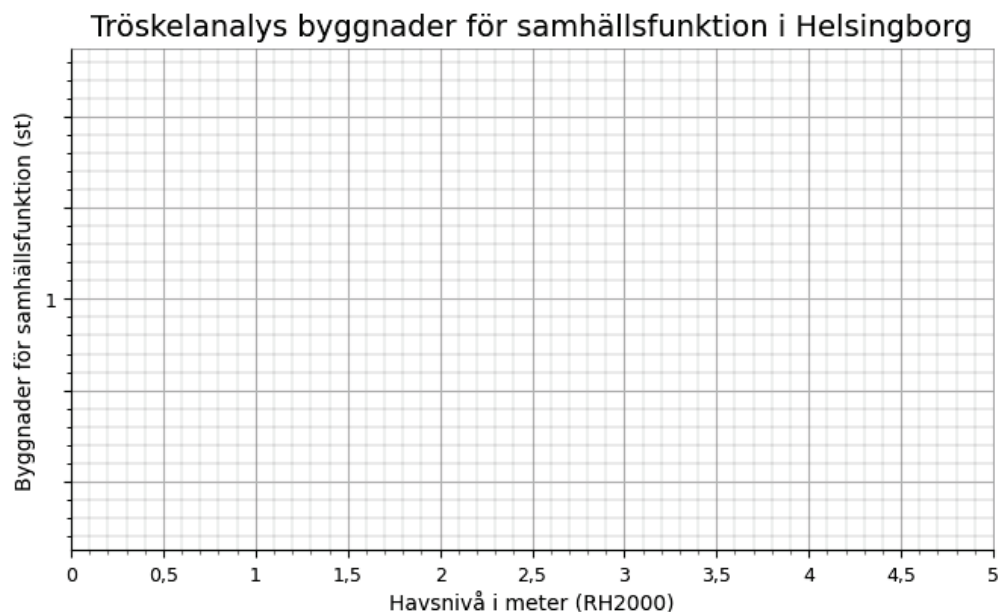
Figur 8 Antal byggnader för samhällsfunktion i Helsingborg kommun som riskerar att översvämmas vid havsnivåer mellan 0-5 m. De samhällsfunktioner som inkluderas i analysen är Sjukhus, Brandstation, Vårdcentral, Kommunhus och Polisstation.
