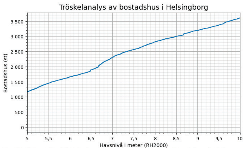
Figur 5 Antalet bostadshus i Helsingborg kommun som riskerar att översvämmas vid havsnivåer mellan 5-10 m. Bostadshus kan delas in i följande ändamål: Småhus friliggande, Småhus kedjehus, Småhus radhus, Småhus med flera lägenheter och Flerfamiljshus.
