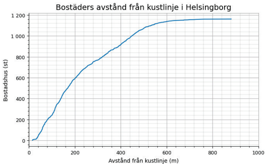
Figur 17 Antal bostadshus inom 1 km från kusten som översvämmas vid havsnivåer <5 m (RH2000) i Helsingborg kommun.
