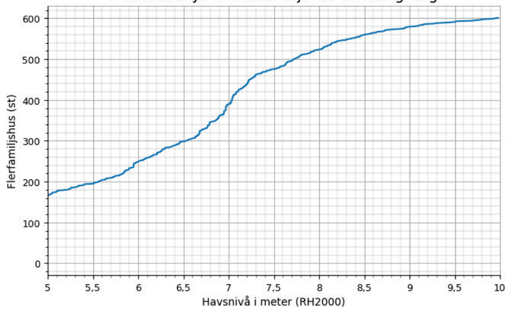
Figur 7 Antalet flerfamiljshus i Helsingborg kommun som riskerar att översvämmas vid havsnivåer mellan 5-10 m.
