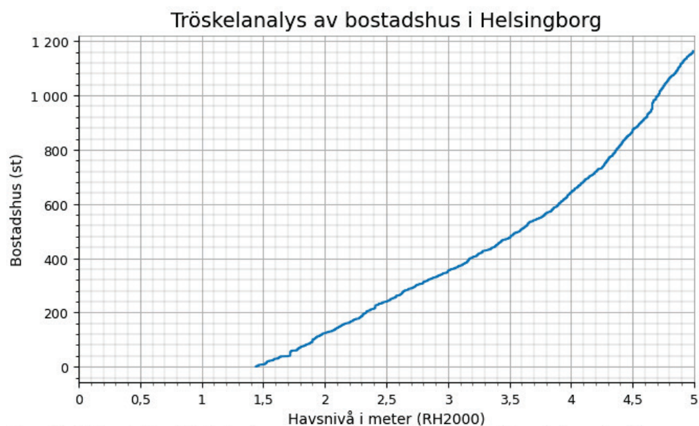
Figur 4 Antalet bostadshus i Helsingborg kommun som riskerar att översvämmas vid havsnivåer mellan 0-5 m. Bostadshus kan delas in i följande ändamål: Småhus friliggande, Småhus kedjehus, Småhus radhus, Småhus med flera lägenheter och Flerfamiljshus.
