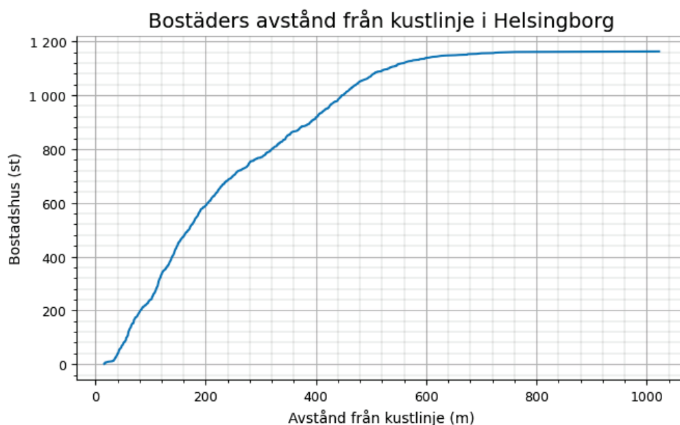
Figur 16 Antal bostadshus på givet avstånd från kusten som översvämmas vid havsnivåer <5 m (RH2000) i Helsingborg kommun. X-axelns utbredning bestäms av det maximala avståndet från kustlinjen till ett bostadshus som översvämmas vid <5 m (RH2000).
