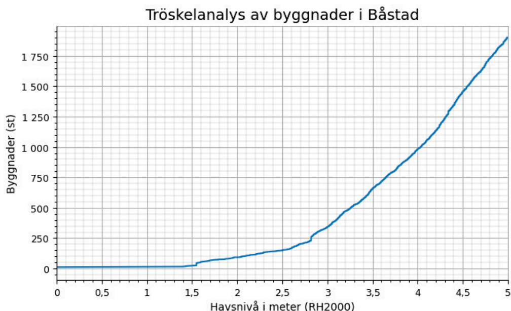
Figur 3 Antalet byggnader i Båstad kommun som riskerar att översvämmas vid havsnivåer mellan 0-5 m. Byggnader består av följande objektstyper: Bostad, Industri, Samhällsfunktion, Verksamhet, Ekonomibyggnad, Komplementbyggnad och Övrig byggnad.
