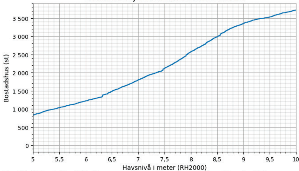
Figur 5 Antalet bostadshus i Båstad kommun som riskerar att översvämmas vid havsnivåer mellan 5-10 m. Bostadshus kan delas in i följande ändamål: Småhus friliggande, Småhus kedjehus, Småhus radhus, Småhus med flera lägenheter och Flerfamiljshus.
