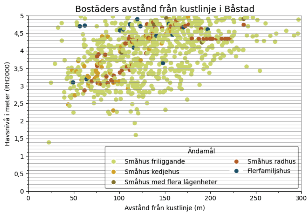
Figur 21 Samband mellan tröskelnivå för havsöversvämning, avstånd från kustlinjen upp till 300 m och ändamålet för bostadshus i Båstad kommun.
