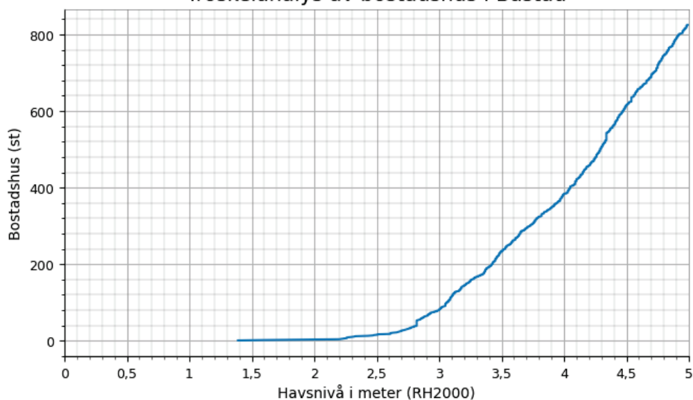
Figur 4 Antalet bostadshus i Båstad kommun som riskerar att översvämmas vid havsnivåer mellan 0-5 m. Bostadshus kan delas in i följande ändamål: Småhus friliggande, Småhus kedjehus, Småhus radhus, Småhus med flera lägenheter och Flerfamiljshus.
