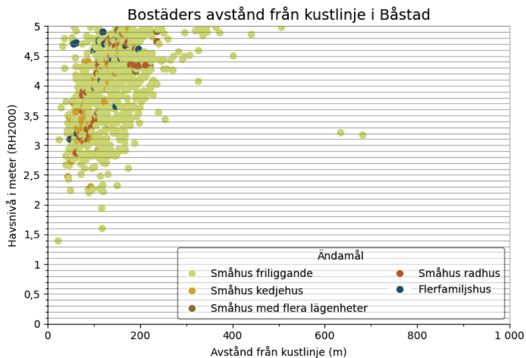
Figur 20 Samband mellan tröskelnivå för havsöversvämnning, avstånd från kustlinjen upp till 1 km och ändamålet för bostadshus i Båstad kommun.
