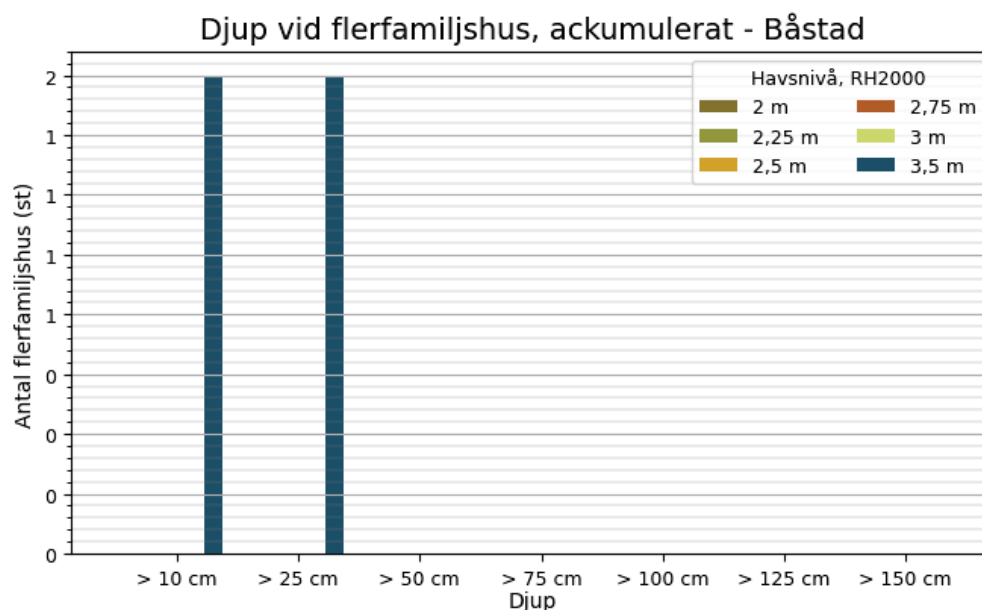
Figur 15 Samband i Båstad kommun mellan havsnivå och antalet flerfamiljshus som översvämmas med ett givet vattendjup eller mer. Förutsätter att havsnivån varar tillräckligt länge för att maximalt potentiellt översvämningsdjup ska hinna nås.
