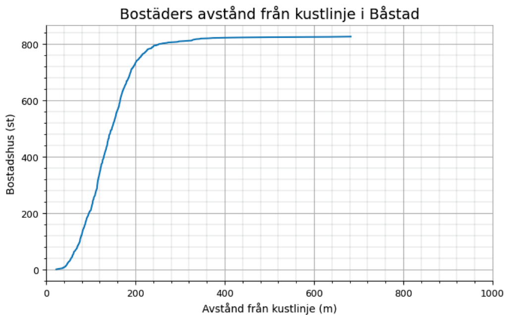
Figur 17 Antal bostadshus inom 1 km från kusten som översvämmas vid havsnivåer <5 m (RH2000) i Båstad kommun.
