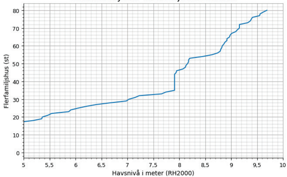
Figur 7 Antalet flerfamiljshus i Båstad kommun som riskerar att översvämmas vid havsnivåer mellan 5-10 m.
