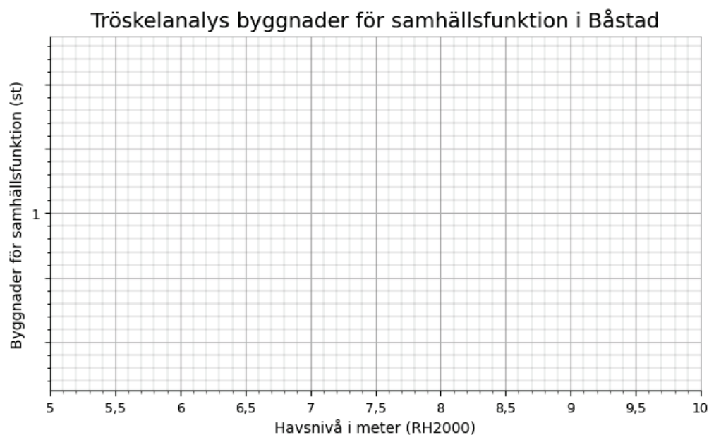
Figur 9 Antal byggnader för samhällsfunktion i Båstad kommun som riskerar att översvämmas vid havsnivåer mellan 5-10 m. De samhällsfunktioner som inkluderas i analysen är Sjukhus, Brandstation, Vårdcentral, Kommunhus och Polisstation.
