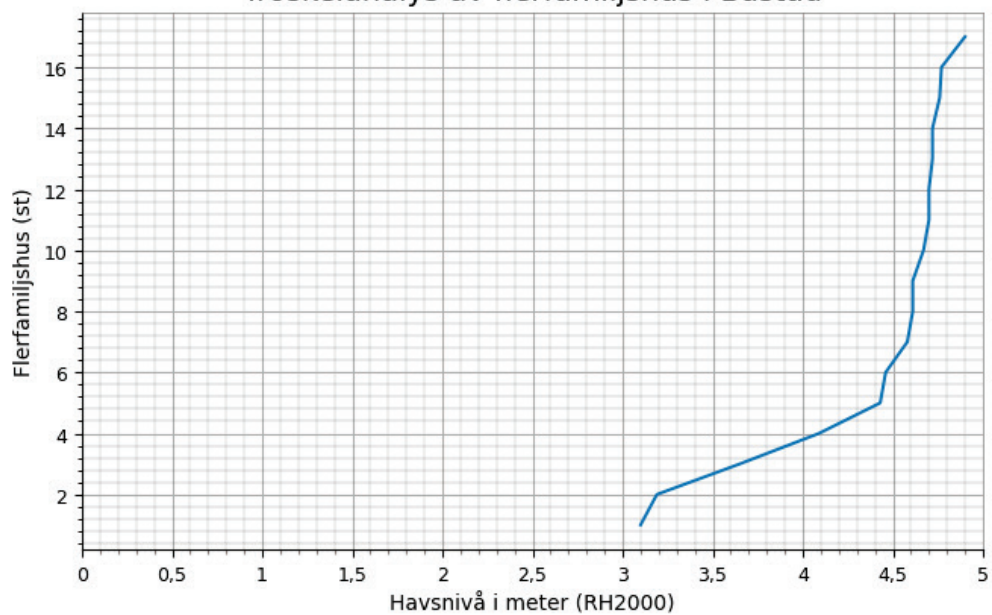
Figur 6 Antalet flerfamiljshus i Båstad kommun som riskerar att översvämmas vid havsnivåer mellan 0-5 m.
