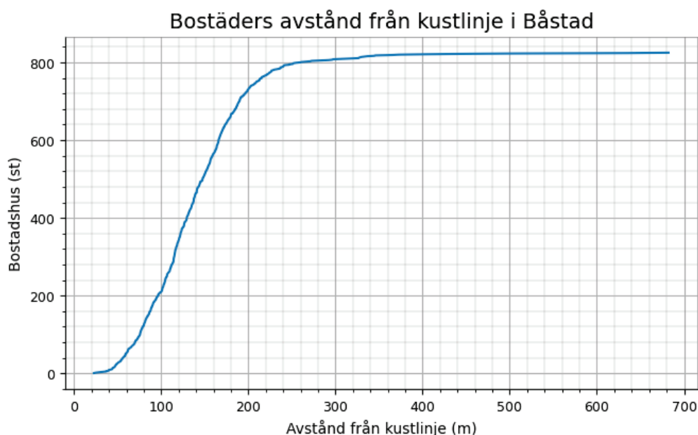
Figur 16 Antal bostadshus på givet avstånd från kusten som översvämmas vid havsnivåer <5 m (RH2000) i Båstad kommun. X-axelns utbredning bestäms av det maximala avståndet från kustlinjen till ett bostadshus som översvämmas vid <5 m (RH2000).
