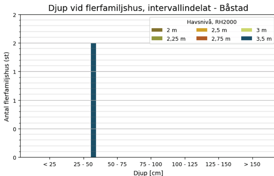
Figur 14 Samband i Båstad kommun mellan havsnivå och antalet flerfamiljshus som drabbas av översvämning, indelat i intervall för översvämningsdjup vid bostaden. Förutsätter att havsnivån varar tillräckligt länge för att maximalt potentiellt översvämningsdjup ska nås.
