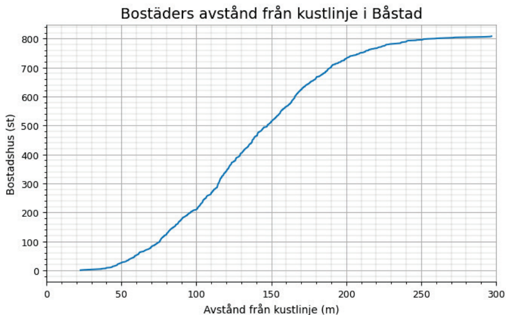
Figur 18 Antal bostadshus inom 300 m från kusten som översvämmas vid havsnivåer <5 m (RH2000) i Båstad kommun.
