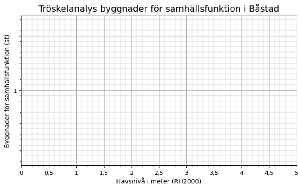
Figur 8 Antal byggnader för samhällsfunktion i Båstad kommun som riskerar att översvämmas vid havsnivåer mellan 0-5 m. De samhällsfunktioner som inkluderas i analysen är Sjukhus, Brandstation, Vårdcentral, Kommunhus och Polisstation.
