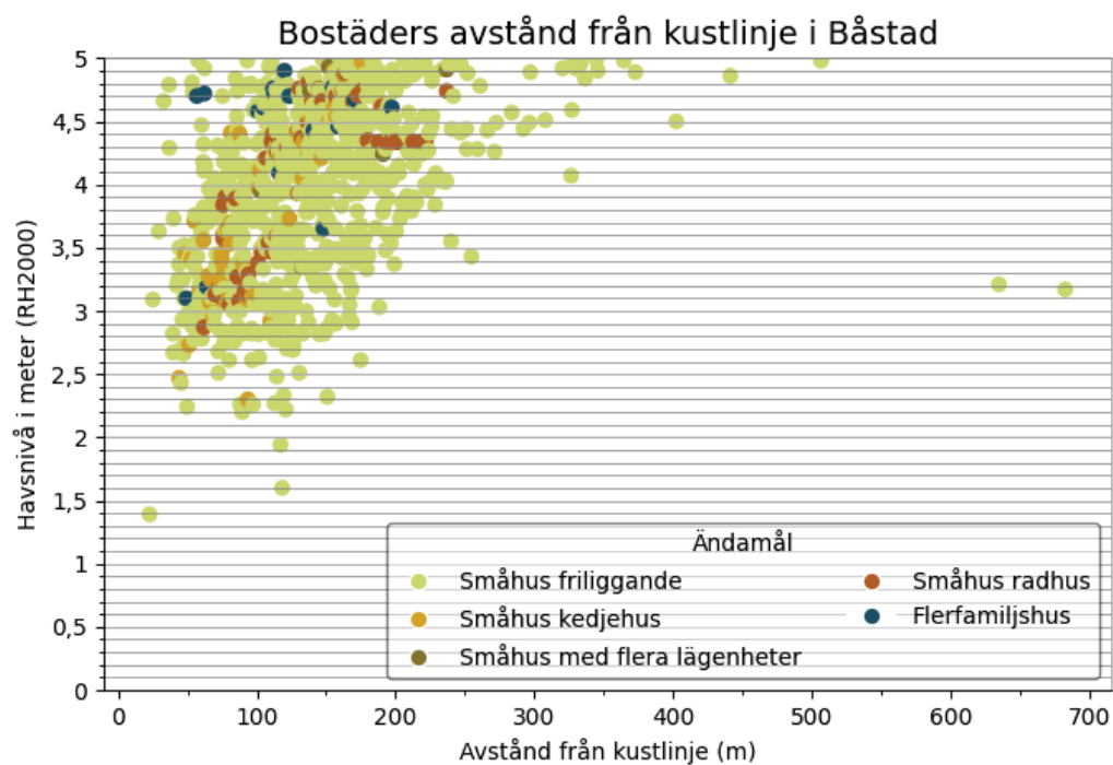
Figur 19 Samband mellan tröskelnivå för havsöversvämnning, avstånd från kustlinjen och ändamålet för bostadshus i Båstad kommun. X-axelns utbredning bestäms av det maximala avståndet från kust till ett bostadshus som översvämmas vid <5 m (RH2000).
