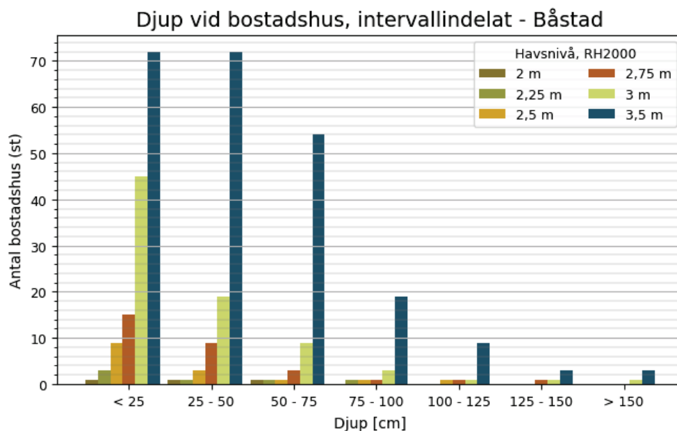
Figur 12 Samband i Båstad kommun mellan havsnivå och antalet bostadshus som drabbas av översvämnning, indelat i intervall för översvämningsdjup vid bostad. Förutsätter att havsnivån varar tillräckligt länge för att maximalt potentiellt översvämningsdjup ska nås.
