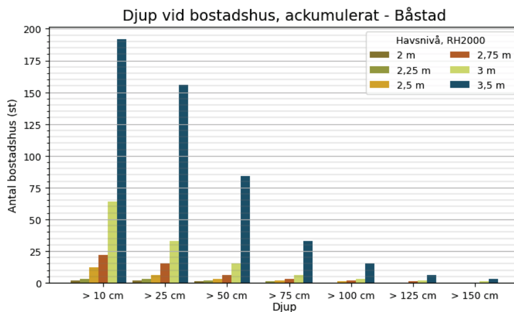
Figur 13 Samband i Båstad kommun mellan havsnivå och antalet bostadshus som översvämmas med ett givet vattendjup eller mer. Förutsätter att havsnivån varar tillräckligt länge för att maximalt potentiellt översvämningsdjup ska hinna nås.
