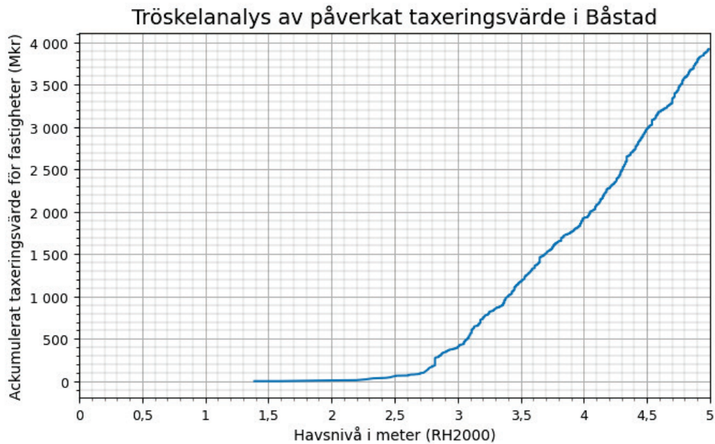
Figur 10 Det ackumulerade taxerade värdet (år 2023) för bostäder i Båstad kommun som riskerar att översvämmas vid havsnivåer mellan 0-5 m. Taxeringsvärdet inkluderar både tomtvärde och byggnadsvärde.
