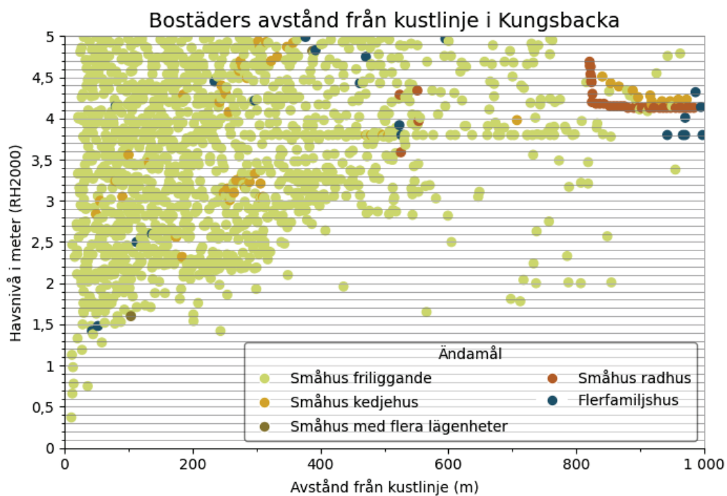
Figur 20 Samband mellan tröskelnivå för havsöversvämning, avstånd från kustlinjen upp till 1 km och ändamålet för bostadshus i Kungsbacka kommun.
