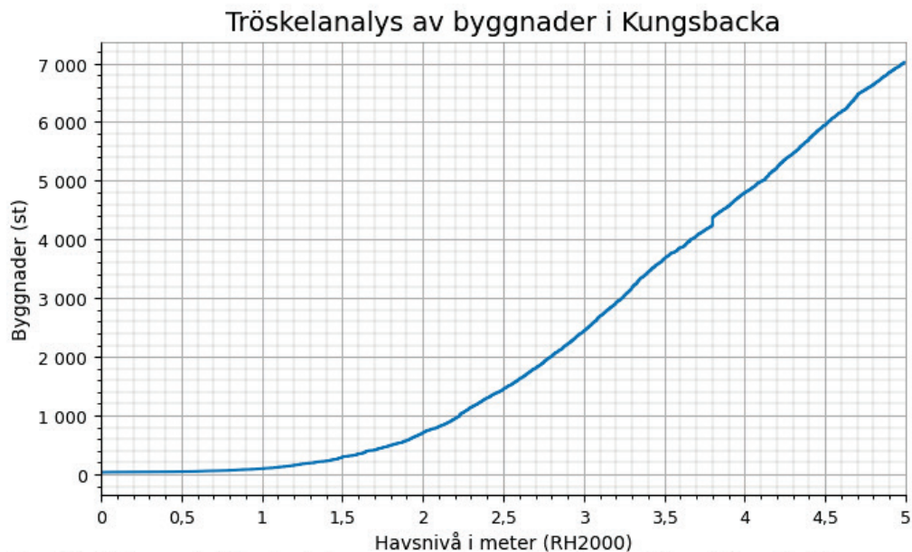
Figur 3 Antalet byggnader i Kungsbacka kommun som riskerar att översvämmas vid havsnivåer mellan 0-5 m. Byggnader består av följande objektstyper: Bostad, Industri, Samhällsfunktion, Verksamhet, Ekonomibyggnad, Komplementbyggnad och Övrig byggnad.
