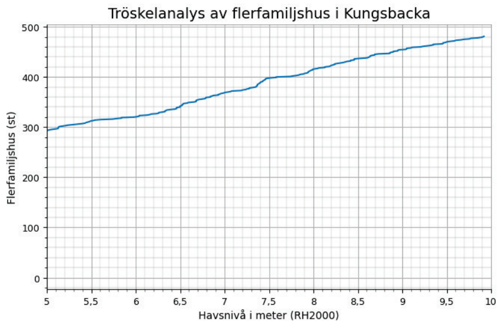
Figur 7 Antalet flerfamiljshus i Kungsbäcka kommun som riskerar att översvämmas vid havsnivåer mellan 5-10 m.
