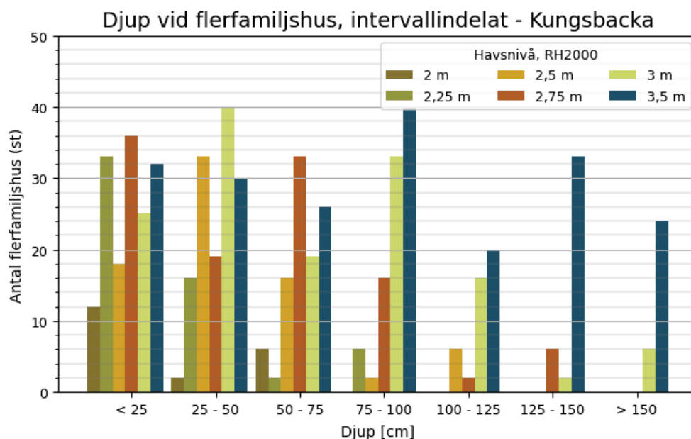
Figur 14 Samband i Kungsbacka kommun mellan havsnivå och antalet flerfamiljshus som drabbas av översvämning, indelat i intervall för översvämningsdjup vid bostaden. Förutsätter att havsnivån varar tillräckligt länge för att maximalt potentiellt översvämningsdjup ska nås.
