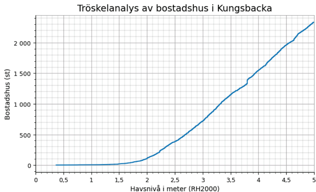
Figur 4 Antalet bostadshus i Kungsbacka kommun som riskerar att översvämmas vid havsnivåer mellan 0-5 m. Bostadshus kan delas in i följande ändamål: Småhus friliggande, Småhus kedjehus, Småhus radhus, Småhus med flera lägenheter och Flerfamiljshus.
