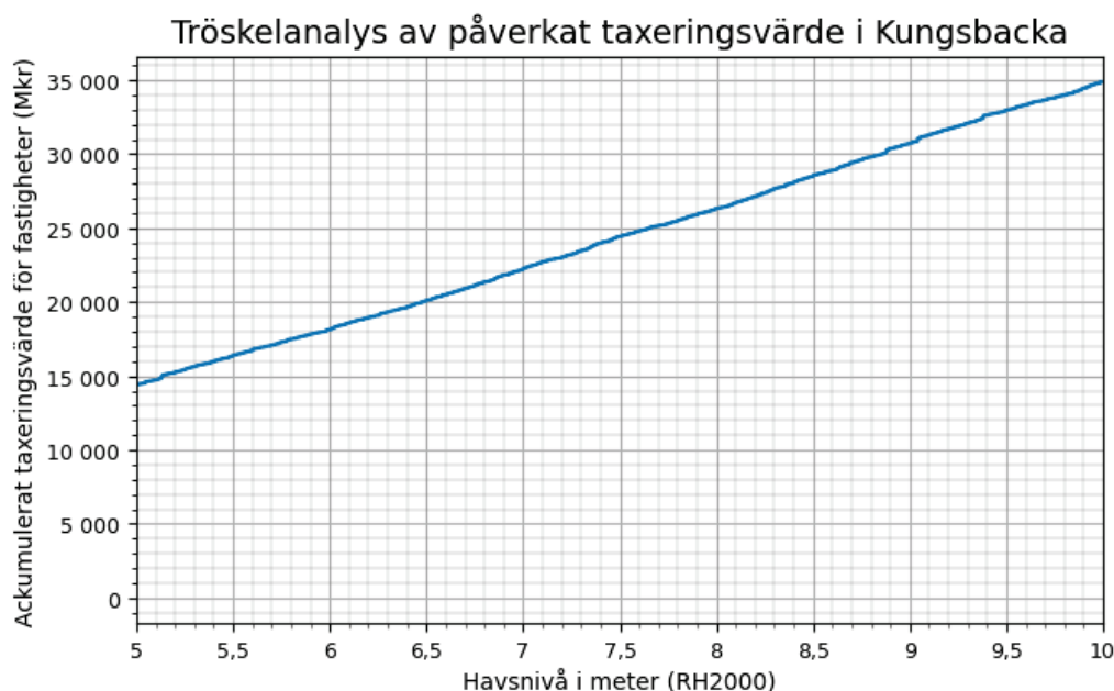
Figur 11 Det ackumulerade taxerade värdet (år 2023) för bostäder i Kungsbäck kommun som riskerar att översvämmas vid havsnivåer mellan 5-10 m. Taxeringsvärdet inkluderar både tomtvärde och byggnadsvärde.
