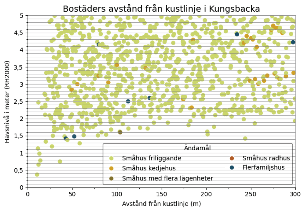
Figur 21 Samband mellan tröskelnivå för havsöversvämning, avstånd från kustlinjen upp till 300 m och ändamålet för bostadshus i Kungsbacka kommun.
