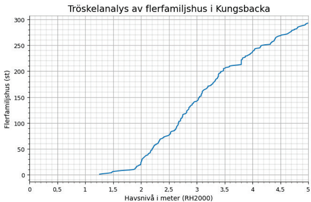
Figur 6 Antalet flerfamiljshus i Kungsbäcka kommun som riskerar att översvämmas vid havsnivåer mellan 0-5 m.
