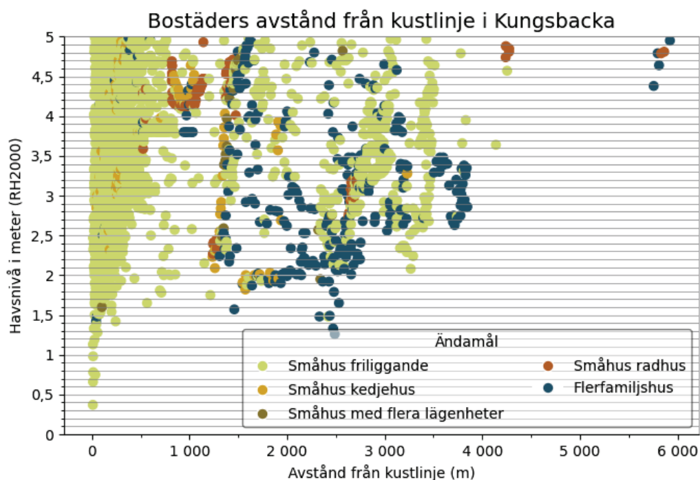
Figur 19 Samband mellan tröskelnivå för havsöversvämning, avstånd från kustlinjen och ändamålet för bostadshus i Kungsbacka kommun. X-axelns utbredning bestäms av det maximala avståndet från kust till ett bostadshus som översvämmas vid <5 m (RH2000).
