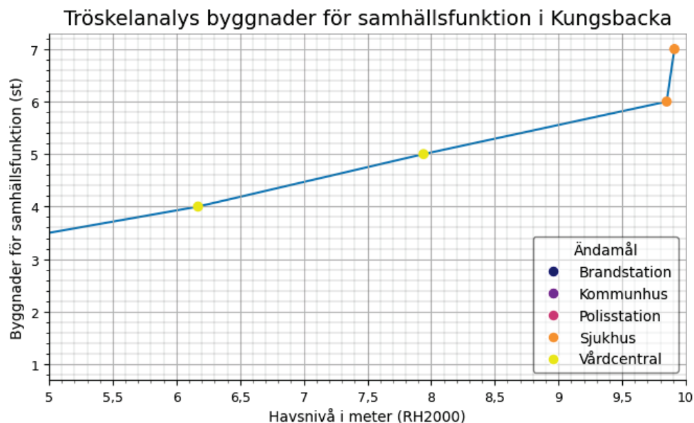
Figur 9 Antal byggnader för samhällsfunktion i Kungsbacka kommun som riskerar att översvämmas vid havsnivåer mellan 5-10 m. De samhällsfunktioner som inkluderas i analysen är Sjukhus, Brandstation, Vårdcentral, Kommunhus och Polisstation.
