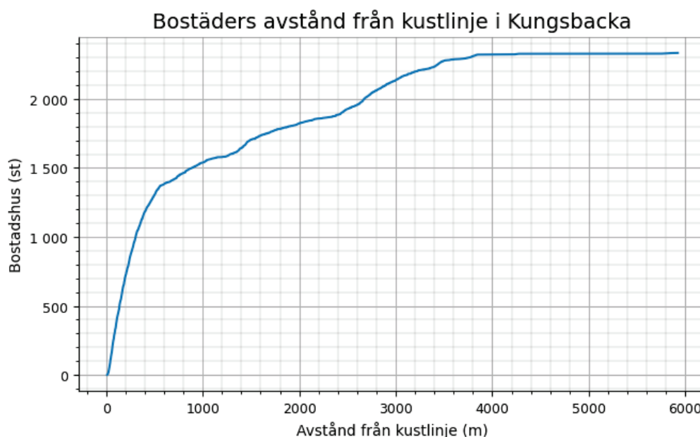
Figur 16 Antal bostadshus på givet avstånd från kusten som översvämmas vid havsnivåer <5 m (RH2000) i Kungsbacka kommun. X-axelns utbredning bestäms av det maximala avståndet från kustlinjen till ett bostadshus som översvämmas vid <5 m (RH2000).
