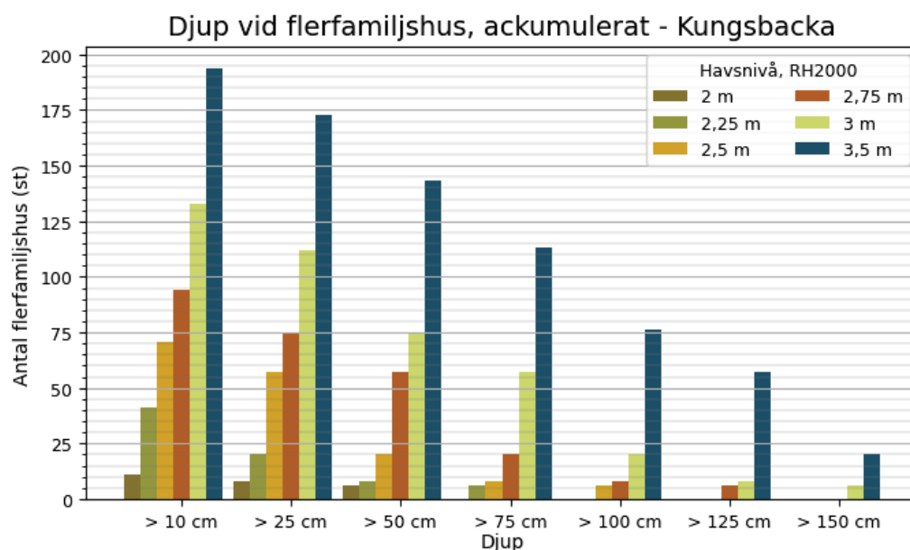
Figur 15 Samband i Kungsbacka kommun mellan havsnivå och antalet flerfamiljshus som översvämmas med ett givet vattendjup eller mer. Förutsätter att havsnivån varar tillräckligt länge för att maximalt potentiellt översvämningsdjup ska hinna nås.
