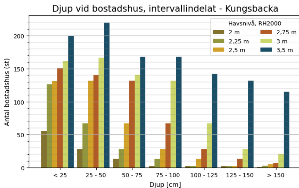
Figur 12 Samband i Kungsbacka kommun mellan havsnivå och antalet bostadshus som drabbas av översvämning, indelat i intervall för översvämningsdjup vid bostad. Förutsätter att havsnivån varar tillräckligt länge för att maximalt potentiellt översvämningsdjup ska nås.
