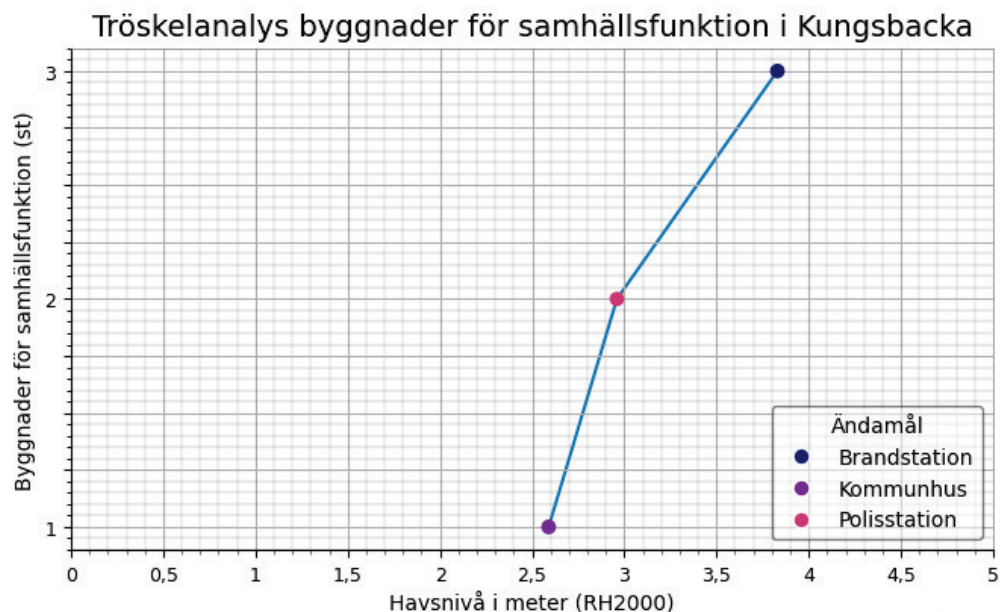
Figur 8 Antal byggnader för samhällsfunktion i Kungsbacka kommun som riskerar att översvämmas vid havsnivåer mellan 0-5 m. De samhällsfunktioner som inkluderas i analysen är Sjukhus, Brandstation, Vårdcentral, Kommunhus och Polisstation.
