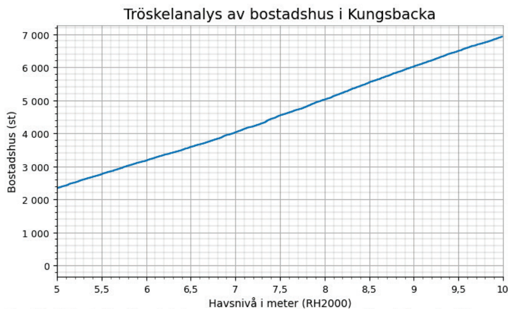
Figur 5 Antalet bostadshus i Kungsbacka kommun som riskerar att översvämmas vid havsnivåer mellan 5-10 m. Bostadshus kan delas in i följande ändamål: Småhus friliggande, Småhus kedjehus, Småhus radhus, Småhus med flera lägenheter och Flerfamiljshus.
