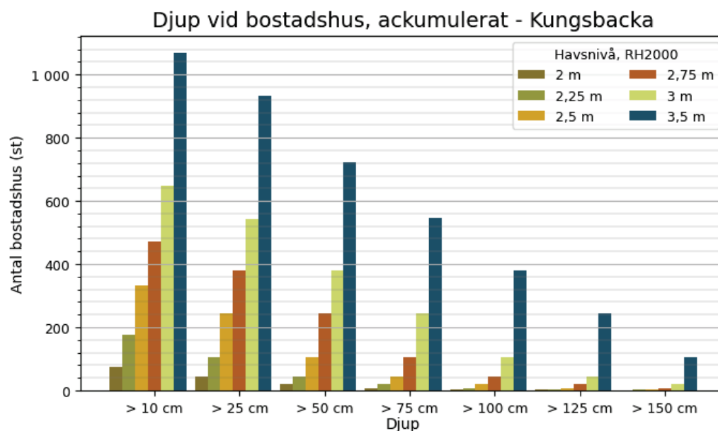
Figur 13 Samband i Kungsbacka kommun mellan havsnivå och antalet bostadshus som översvämmas med ett givet vattendjup eller mer. Förutsätter att havsnivån varar tillräckligt länge för att maximalt potentiellt översvämningsdjup ska hinna nås.
