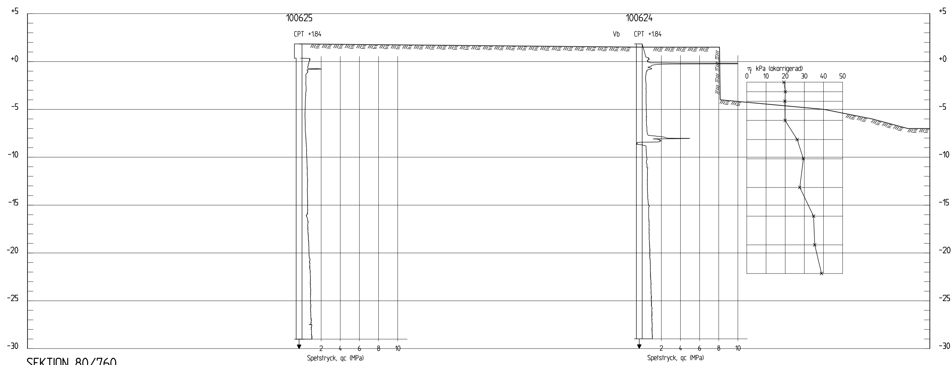
SEKTION 80/760 H 1: 200 L 1: 400
